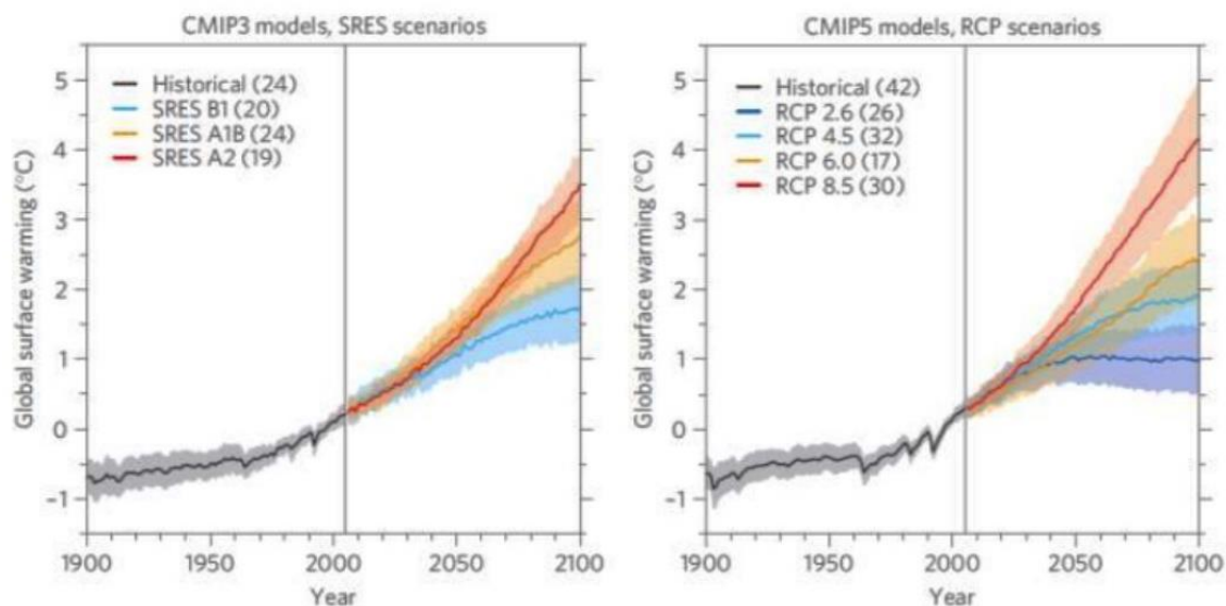
Gráfica 7: Equivalencia de escenarios SRES y RCP desde el punto de vista del forzamiento radiativo (IPCC)
