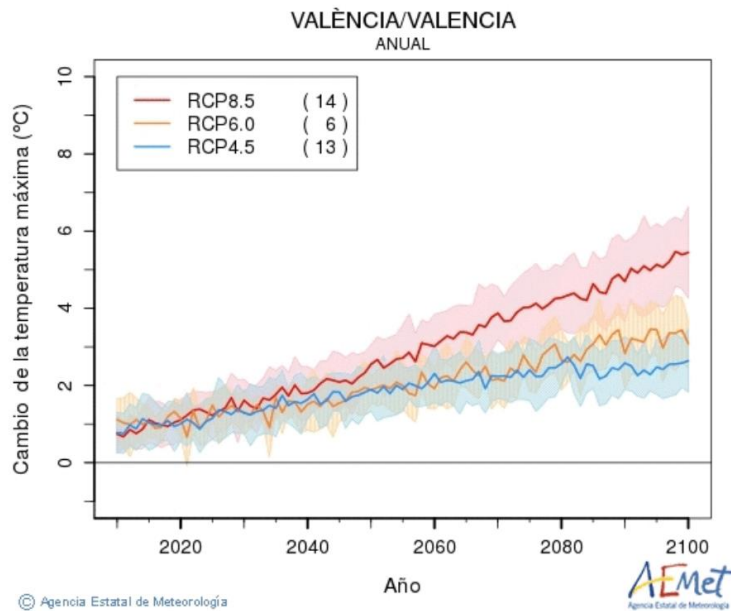
Gráfica 9: Evolución temporal del valor medio anual para la Comunitat Valenciana de las Temperaturas Máximas (°C) según diferentes escenarios fijados por el IPCC.
