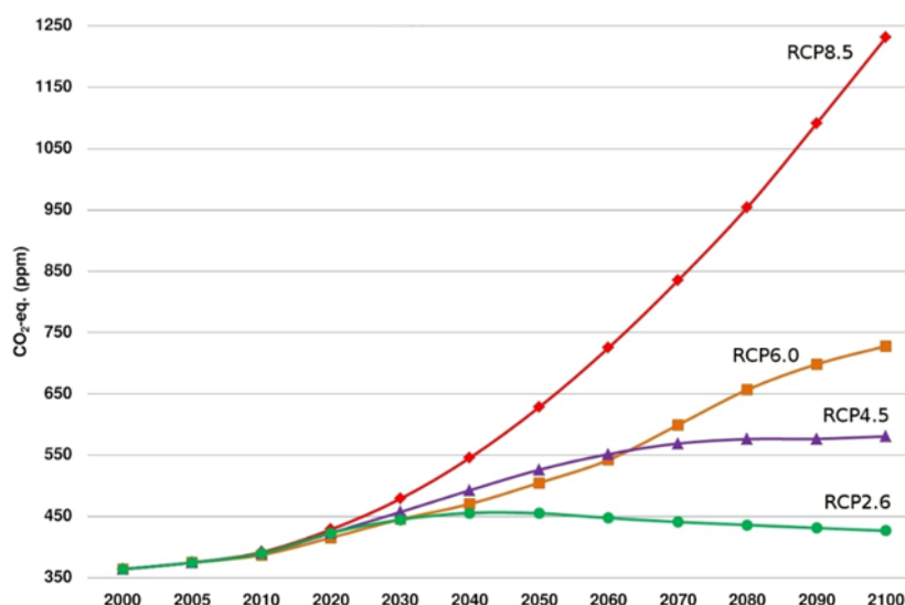
Gráfica 6: Evolución de las concentraciones de gases de efecto invernadero a la atmósfera según los diferentes escenarios RCP.
