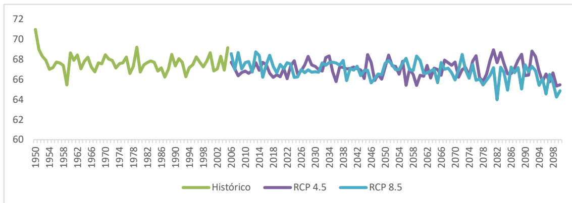
Gráfica 20: Evolución temporal del valor medio anual para la provincia de Valencia de la humedad relativa (%).
