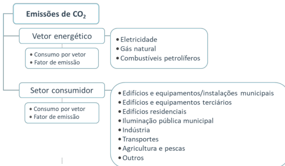
Figura 10 – Representação esquemática da metodologia de cálculo do Inventário de emissões de CO 2 .
