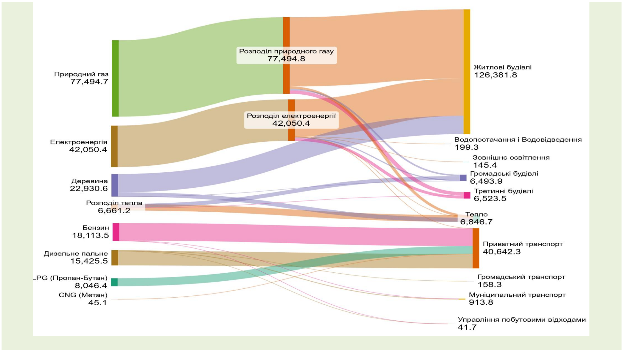
Рис. 3.16. Діаграма Сенкі енергетичної системи Васильківської СТГ станом на 2024 рік
