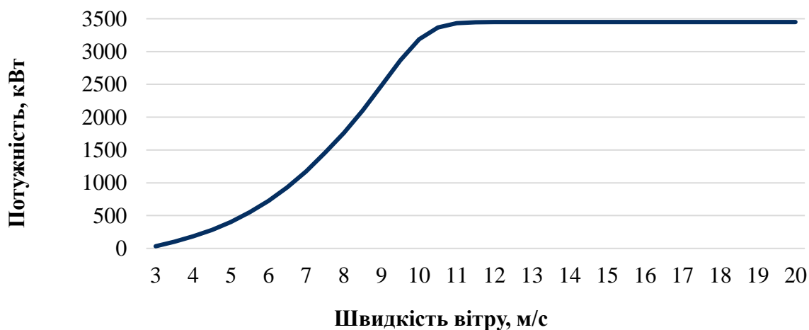
Рис. 1.9. Крива потужності вітротурбіни Vestas V126-3.45.
