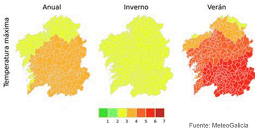
Figura 5. Cambio de la temperatura máxima anual en invierno y en verano en °C. Mostrando las diferencias de valor medio 2061-2090 con respecto a 1971-2000 10
