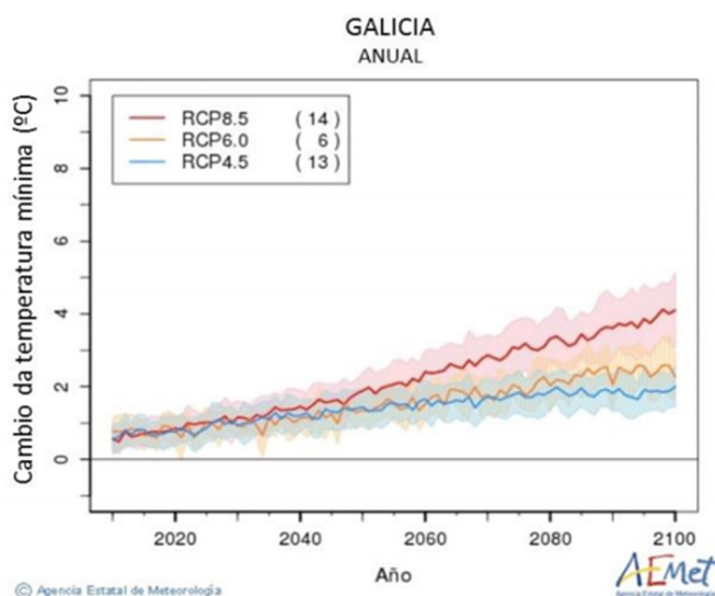
Figura 8_ Cambio en la temperatura mínima para Galicia en el próximo siglo.
