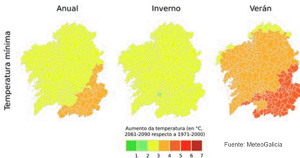
Figura 9_Evolución prevista para la temperatura mínima en Galicia en los años 2061-2090 con respecto a 1971-2000
