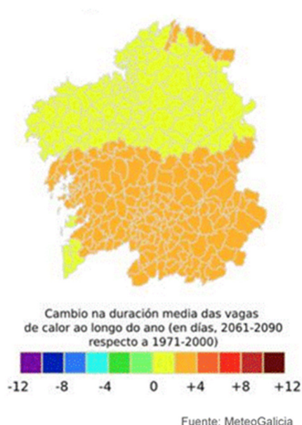
Figura 7. Cambio en la duración promedio de las olas de calor a largo plazo para la comunidad autónoma de Galicia
