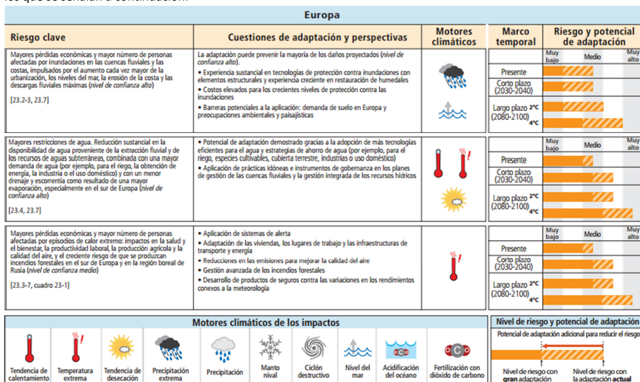
Figura 13_Riesgos clave identificados para el continente europeo en el quinto informe del IPCC
