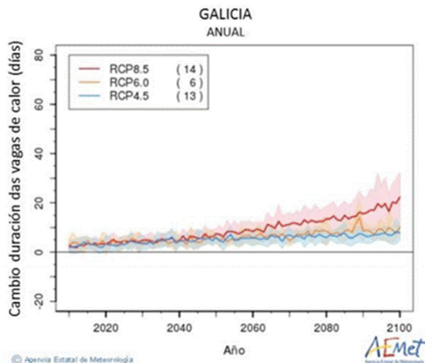
Figura 6. Cambio en la duración de las olas de calor para el próximo siglo en Galicia
