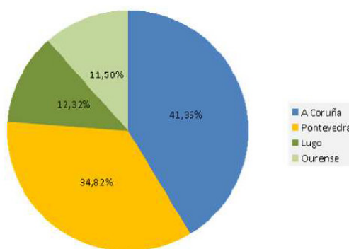
Imagen 8_Distribucion demográfica de Galicia por provincias. Fuente: IGE. Año 2017
