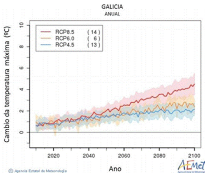
Figura 4. Predicción de la evolución de la temperatura máxima en Galicia.
