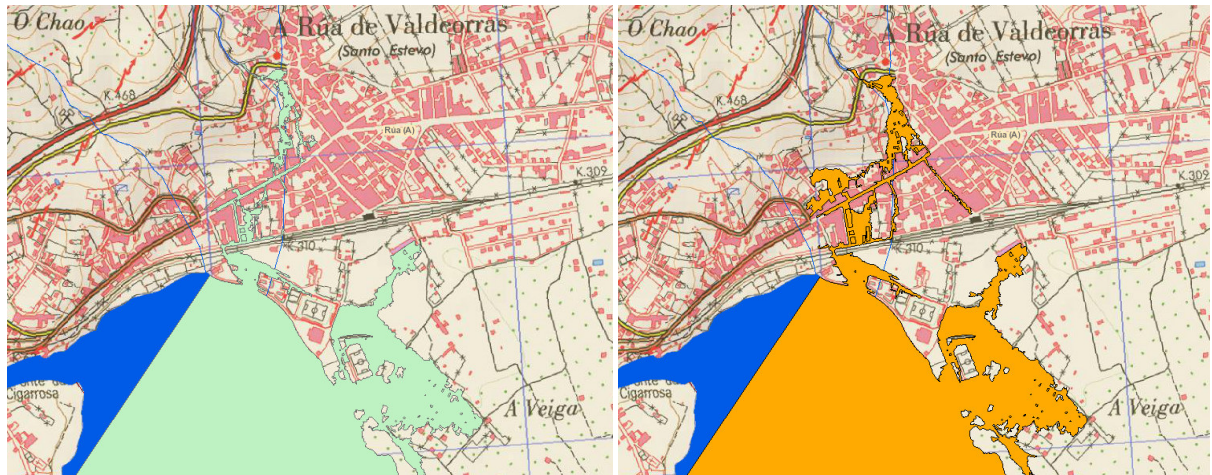
Imagen 15_Mapa de riesgo de inundación de A Rúa. En verde, zonas inundables con alta probabilidad (T=10 años); en naranja, zonas inundables de probabilidad media u ocasional (T= 100 años)
