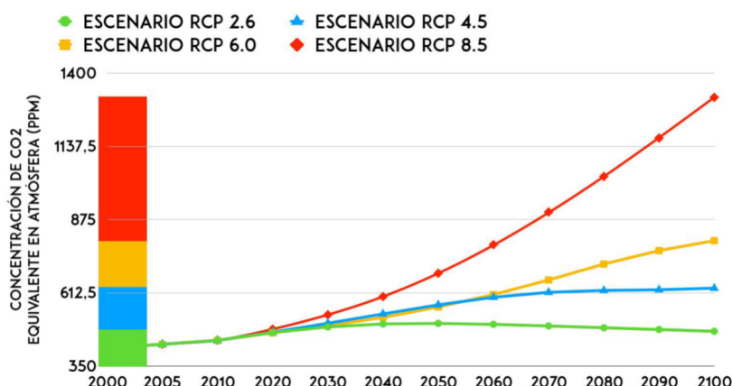
Figura 2_Concentraciones de dióxido de carbono equivalente en la atmósfera según las Trayectorias de Concentraciones Representativas (o RCPs por sus siglas en inglés). Datos: http://www.iiasa.ac.at/web-apps/tnt/RcpDb/dsd?Action=htmlpage&page=compare
