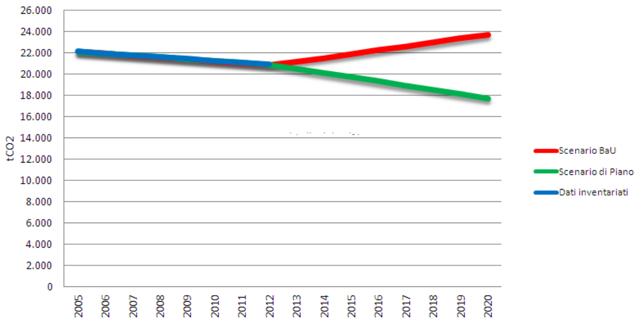
Grafico 16 – Scenario di sviluppo Comune di Pizzighettone
