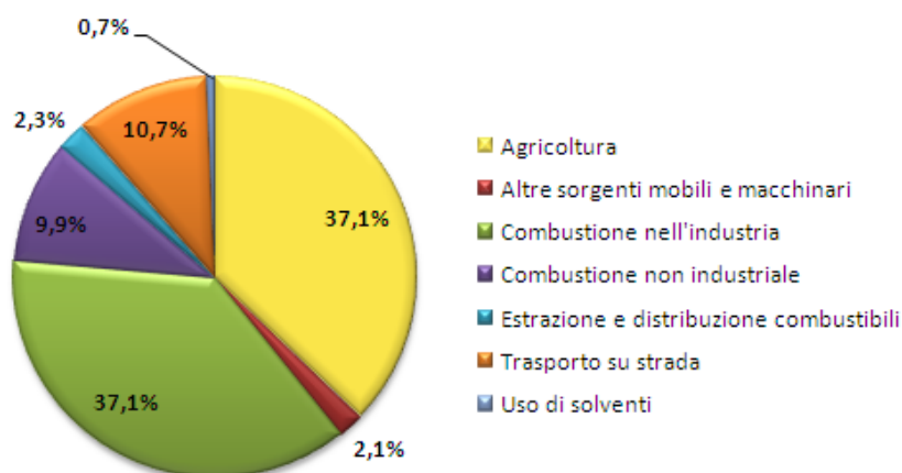
Grafico 6 – Emissioni di CO 2 per settore (INEMAR 2010)
