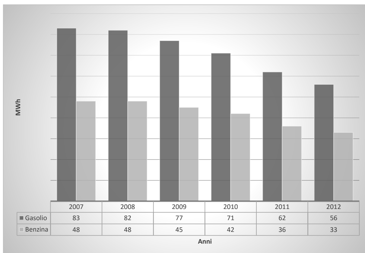
Fig. 22 Consumi del parco veicoli comunale.
