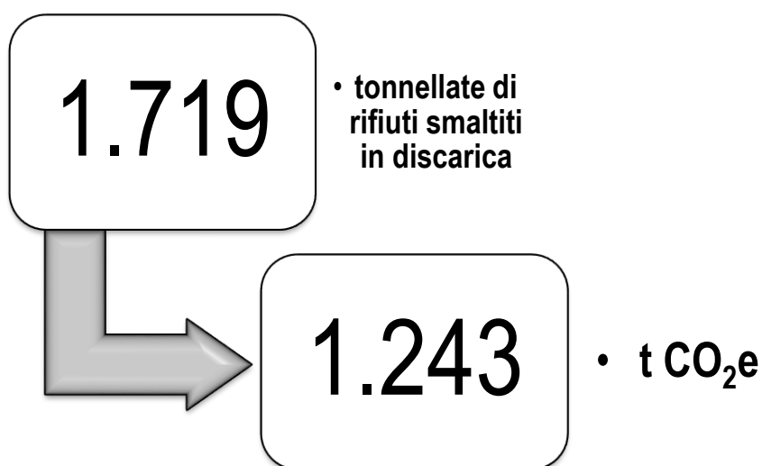
Fig. 36 Quantità rifiuti ed emissioni equivalenti (2007).
