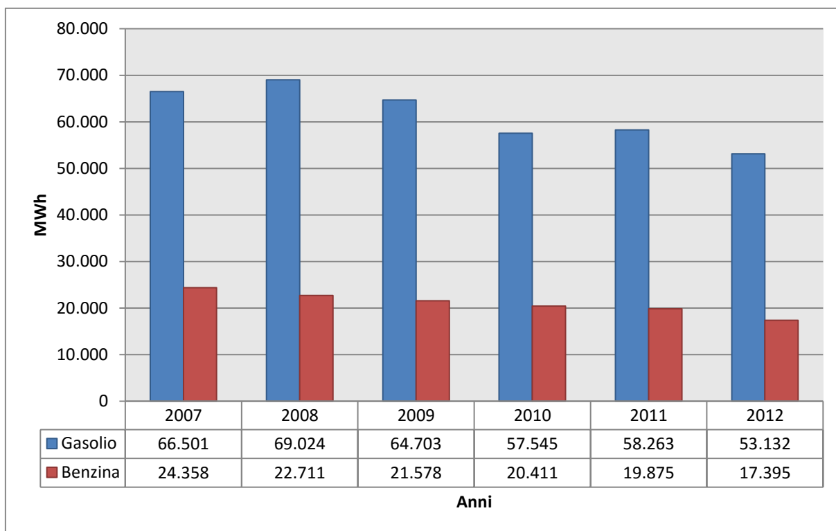
Fig. 30 Consumi nei trasporti privati.
