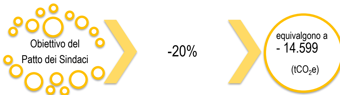
Fig. 42. Obiettivo di riduzione delle emissioni.
