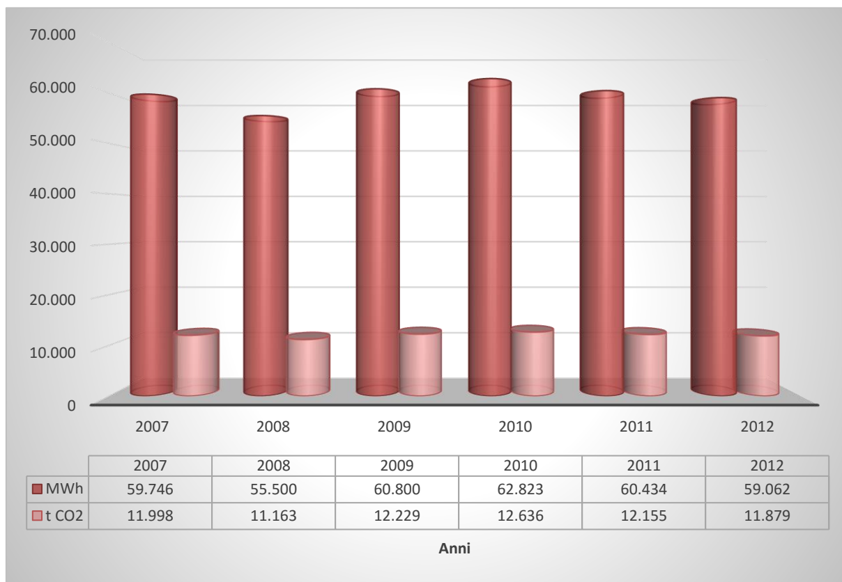
Fig. 25 Consumi ed emissioni di gas metano del territorio comunale.
