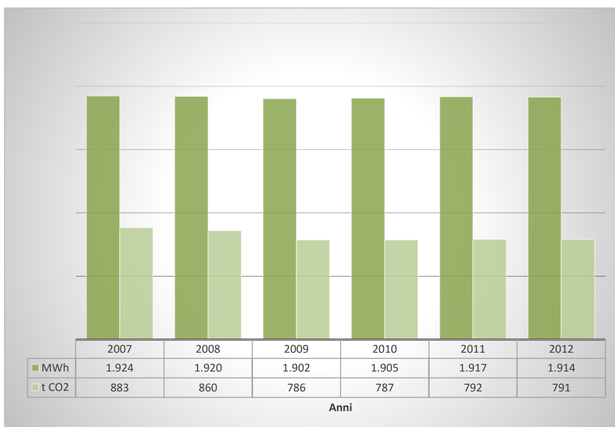
Fig. 23 Consumi ed emissioni dell'illuminazione pubblica.
