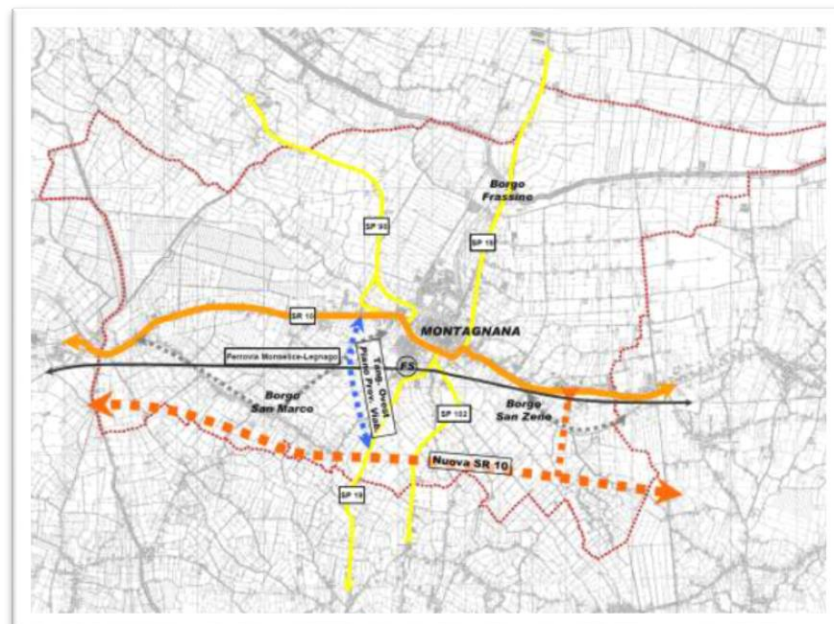
Fig. 10. Sistema della viabilità. (Fonte: Rapporto ambientale Montagnana 2010)
