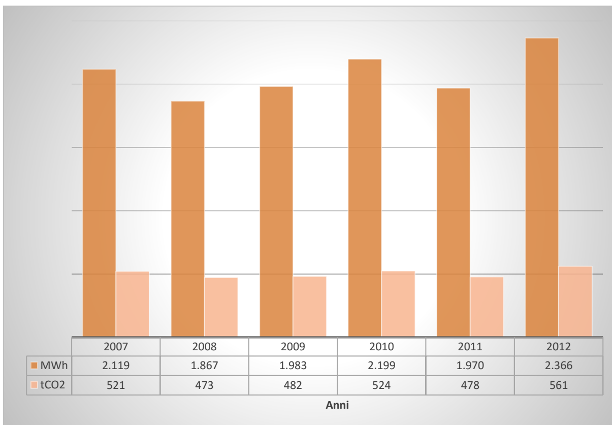
Fig. 21 Consumi ed emissioni degli Edifici comunali
