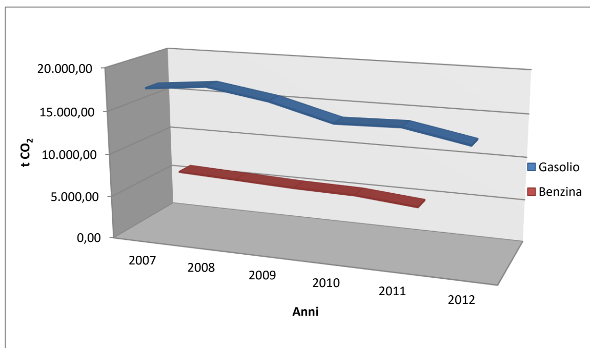
Fig. 31 Emissioni nei trasporti privati.
