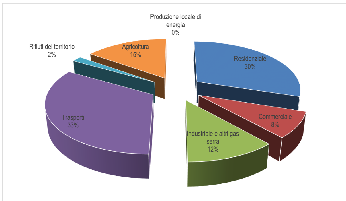
Fig. 17 Emissioni del settore privato per settore (CO 2 ).
