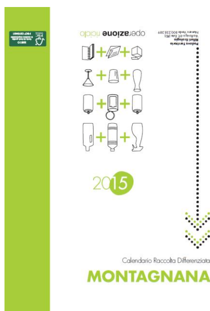
Fig. 33 Calendario raccolta differenziata 2015 (Fonte: http://www.padovasud.it/index.php ).
