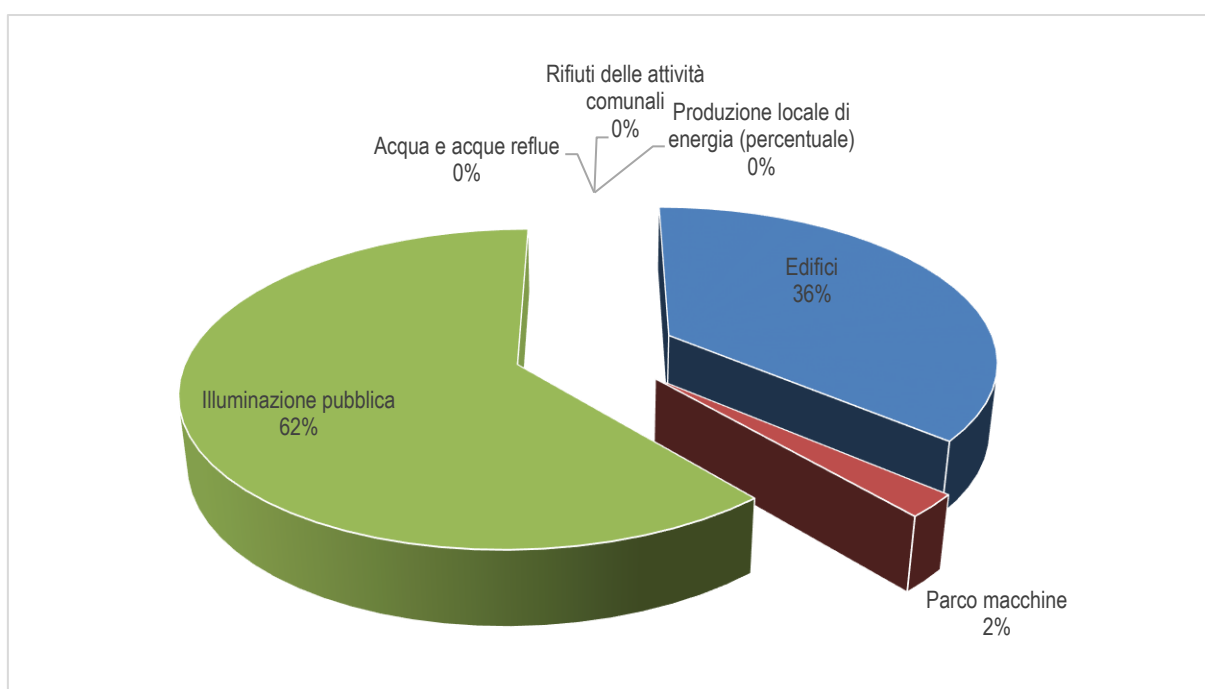
Fig. 20 Dettaglio delle emissioni di CO 2 per settore.
