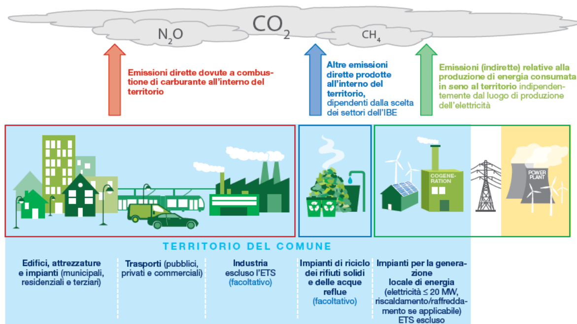
Fig. 11 Divisione delle emissioni per calcolo dell'IBE (Fonte: CoMO 2012)
