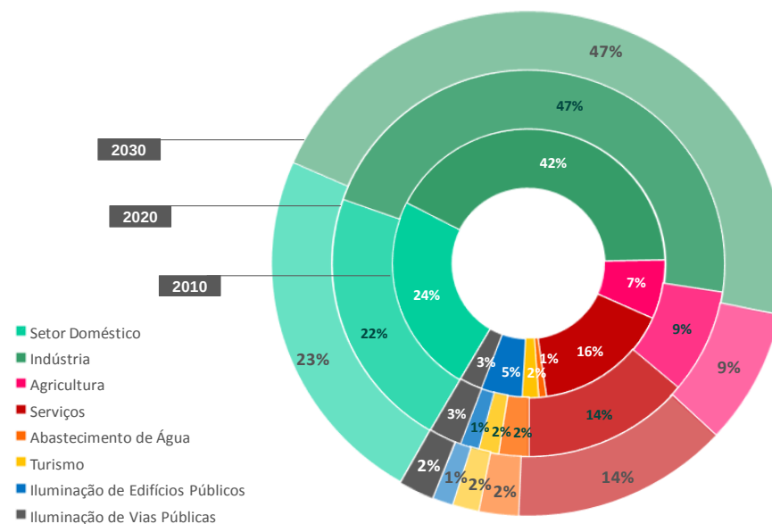
Figura 4 - Consumo de Energia Elétrica por Setor de Atividade em 2010, 2020 e 2030 [%]
