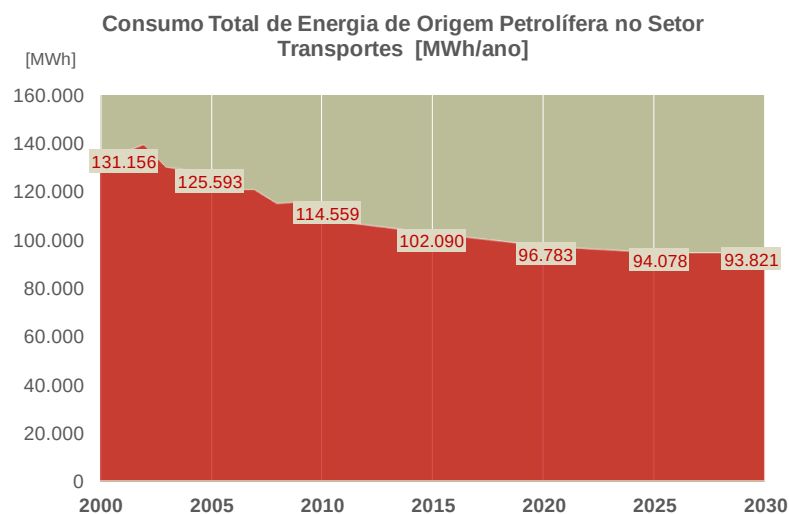
Figura 33 - Consumo Total de Energia de Origem Petrolífera no Setor Transportes
