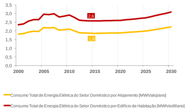
Figura 34 - Consumo Total de Energia Elétrica do Setor Doméstico por Edifício de Habitação e por Alojamento
