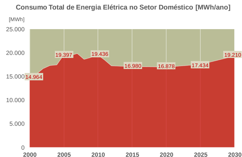
Figura 18 - Consumo Total de Energia Elétrica no Setor Doméstico
