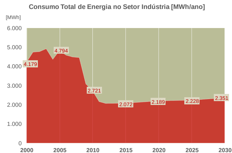
Figura 13 - Consumo Total de Energia no Setor Indústria
