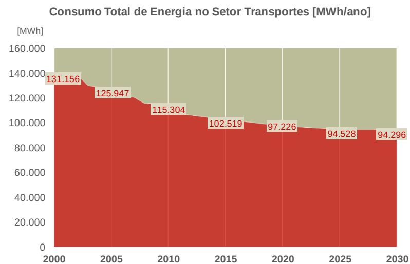
Figura 16 - Consumo Total de Energia no Setor Transportes
