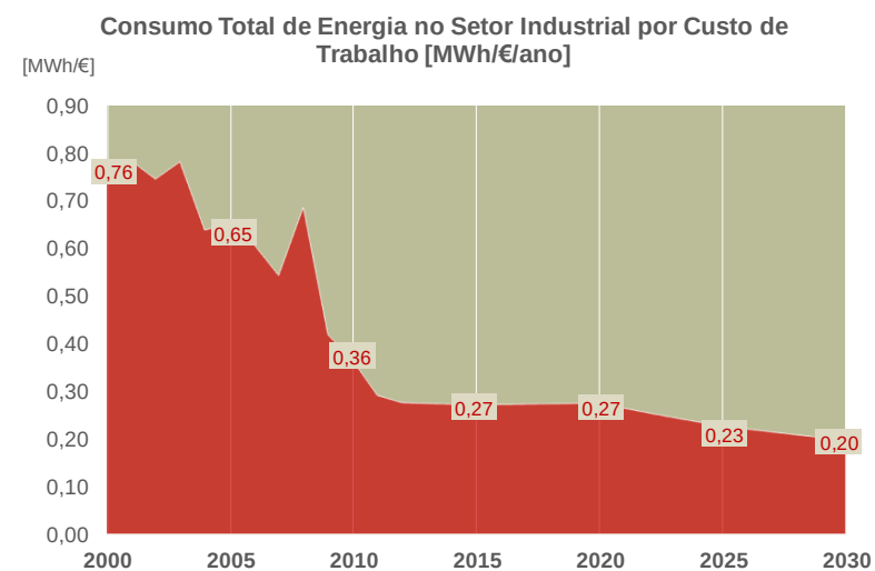
Figura 41 - Consumo Total de Energia no Setor Industrial por Custo de Trabalho
