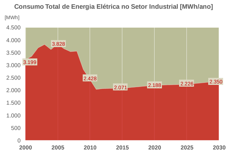
Figura 19 - Consumo de Energia Elétrica no Setor Industrial
