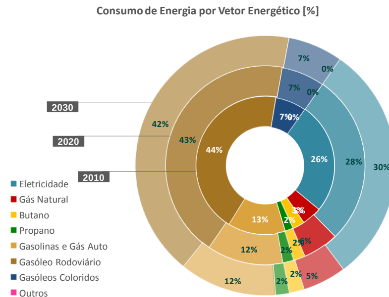
Figura 4 - Consumo de Energia por Vetor Energético em 2010, 2020 e 2030 [%]
