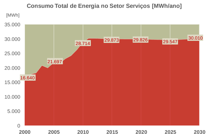
Figura 14 - Consumo Total de Energia no Setor Serviços
