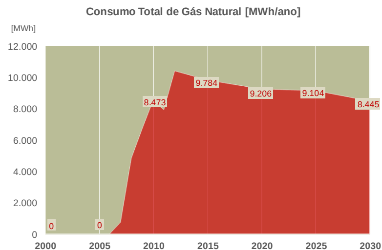
Figura 28 - Consumo Total de Gás Natural
