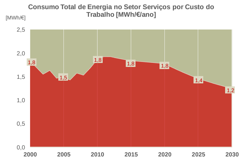
Figura 40 - Consumo Total de Energia no Setor Serviços por Custo do Trabalho
