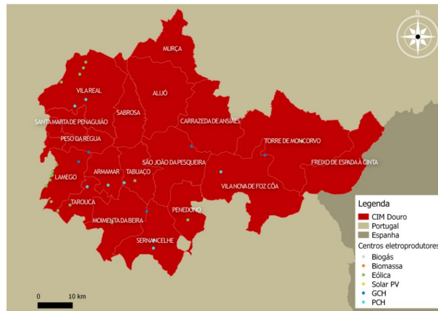
Figura 47 - Centros electroprodutores de base renovável localizados na região de abrangência da CIM Douro (2014)
