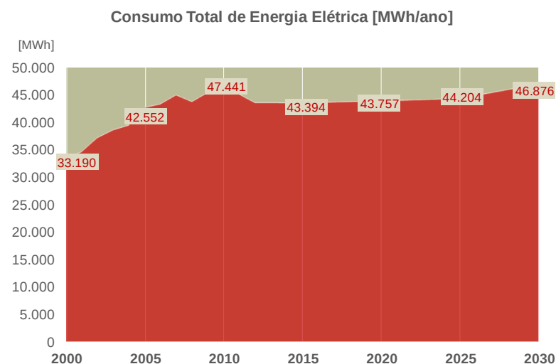
Figura 17 - Consumo Total de Energia Elétrica
