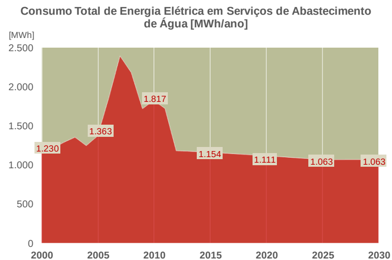
Figura 21 - Consumo Total de Energia Elétrica em Serviços de Abastecimento de Água
