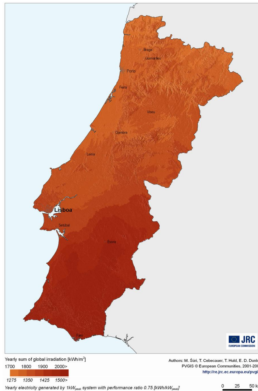
Figura 48 - Irradiação global e potencial máximo de produção de energia elétrica fotovoltaica em Portugal Continental (2010) (Fonte: JRC)
