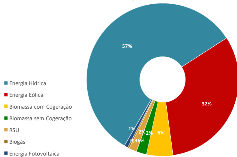
Produção Renovável de Eletricidade em Portugal por Fonte Energética em 2010 [%]
