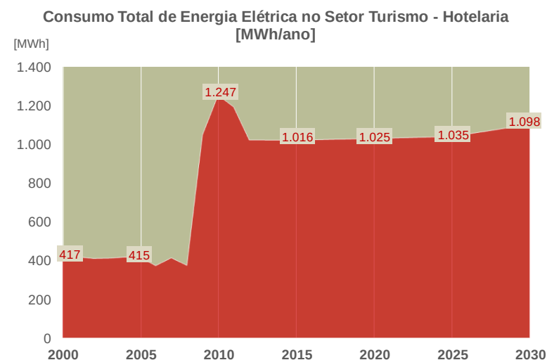
Figura 23 - Consumo Total de Energia Elétrica no Setor Turismo - Hotelaria
