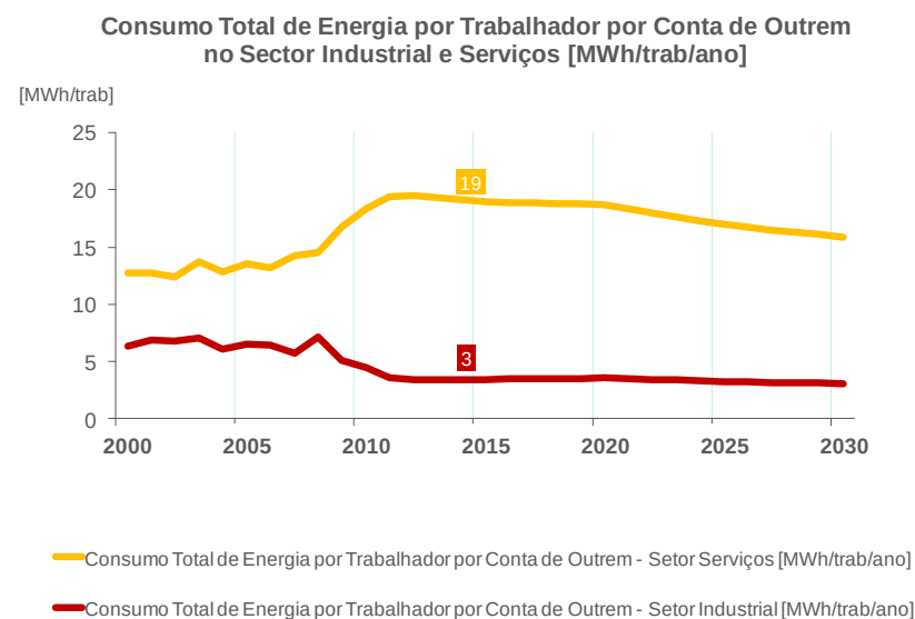
Figura 38 - Consumo Total de Energia por Trabalhador por Conta de Outrem no Setor Industrial e Serviços
