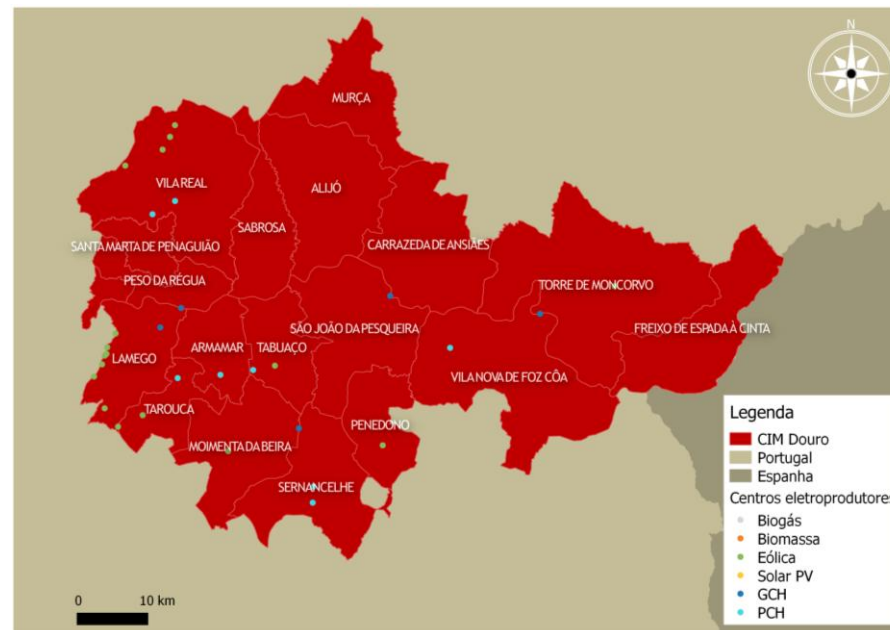
Figura 46 - Centros electroprodutores de base renovável localizados na região de abrangência da CIM Douro (2014)
