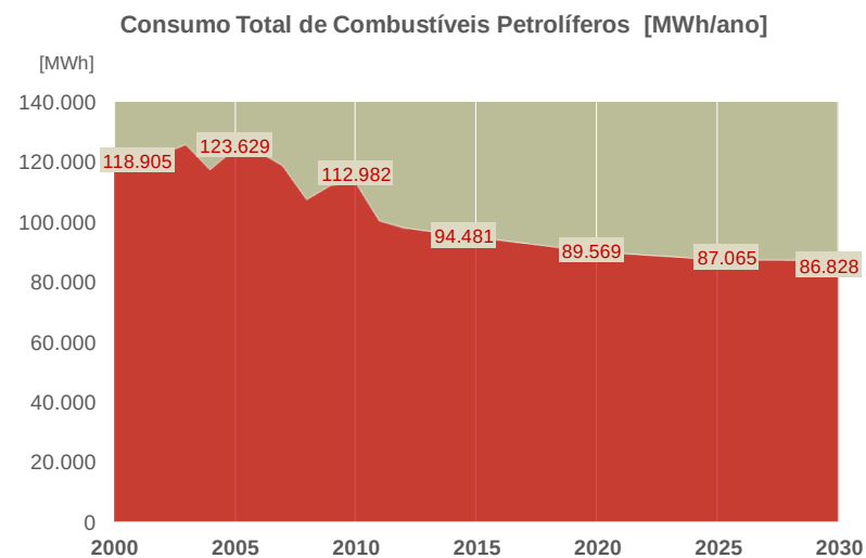
Figura 31 - Consumo Total de Combustíveis Petrolíferos
