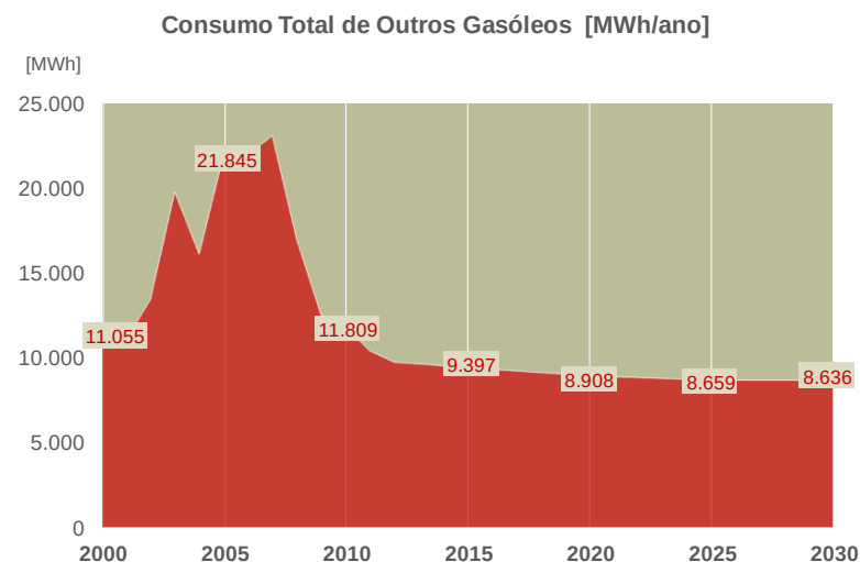
Figura 30 - Consumo Total de Outros Gasóleos
