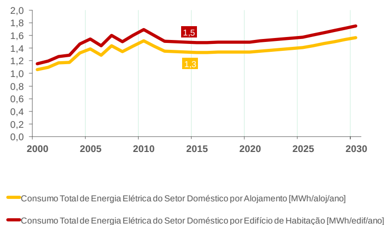
Figura 33 - Consumo Total de Energia Elétrica do Setor Doméstico por Edifício de Habitação e por Alojamento
