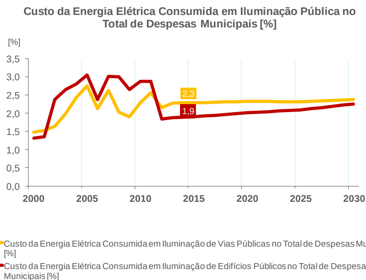
Figura 36 - Custo da Energia Elétrica Consumida em Iluminação Pública no Total de Despesas Municipais
