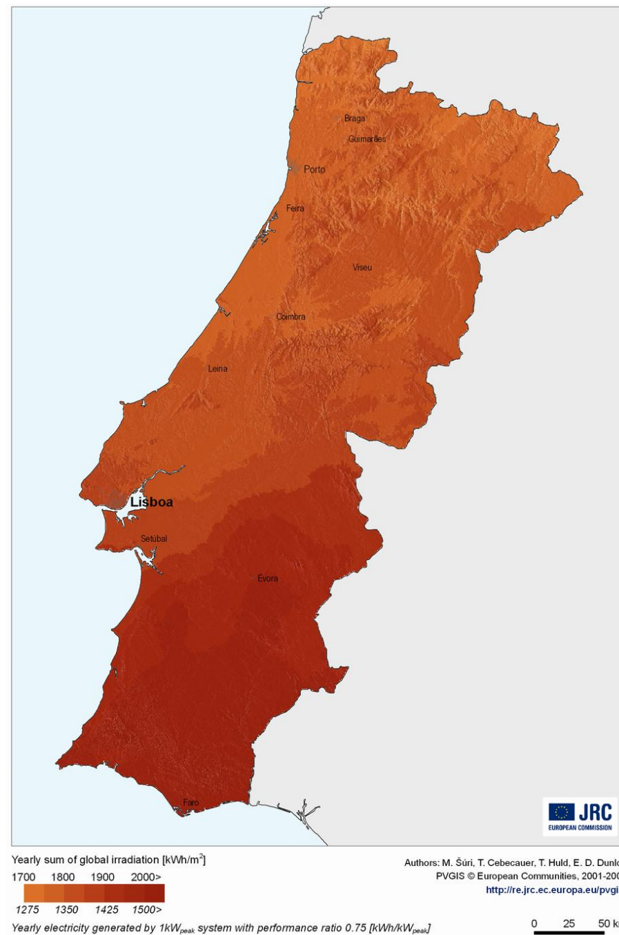
Figura 47 - Irradiação global e potencial máximo de produção de energia elétrica fotovoltaica em Portugal Continental (2010) (Fonte: JRC)
