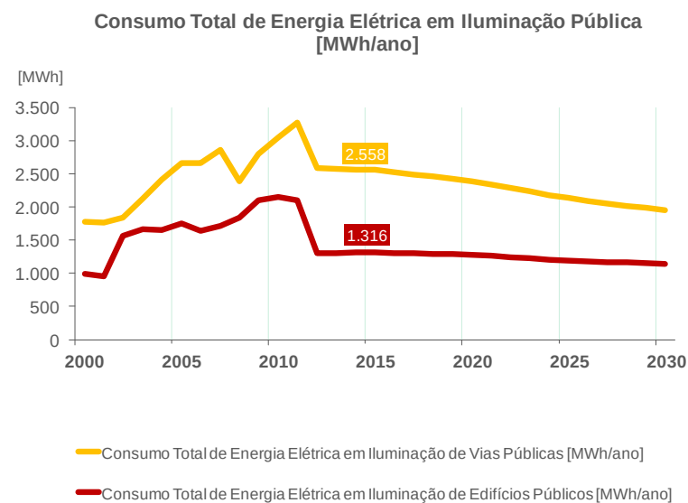
Figura 35 - Consumo Total de Energia Elétrica em Iluminação Pública
