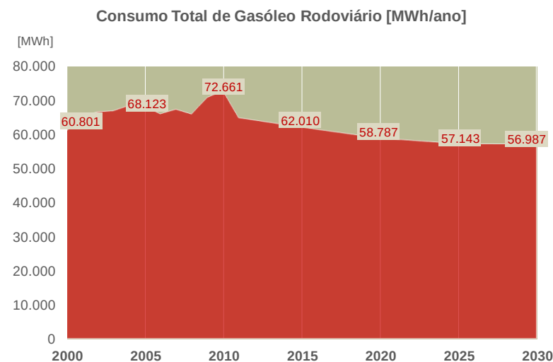
Figura 29 - Total de Gasóleo Rodoviário Vendido
