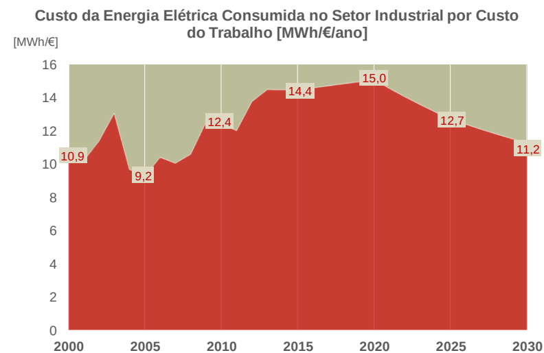
Figura 41 - Custo da Energia Elétrica Consumida no Setor Industrial por Custo do Trabalho
