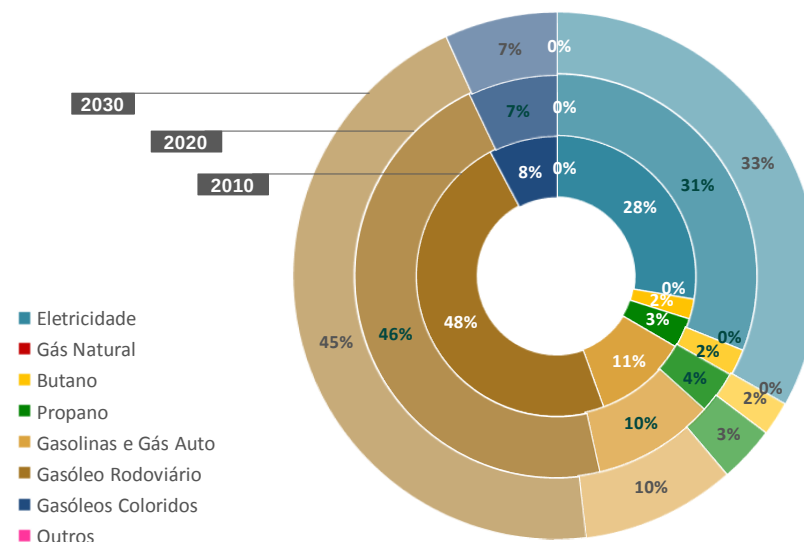
Figura 43 - Emissões de CO 2 por Vetor Energético Consumido em 2010, 2020 e 2030 [%]
