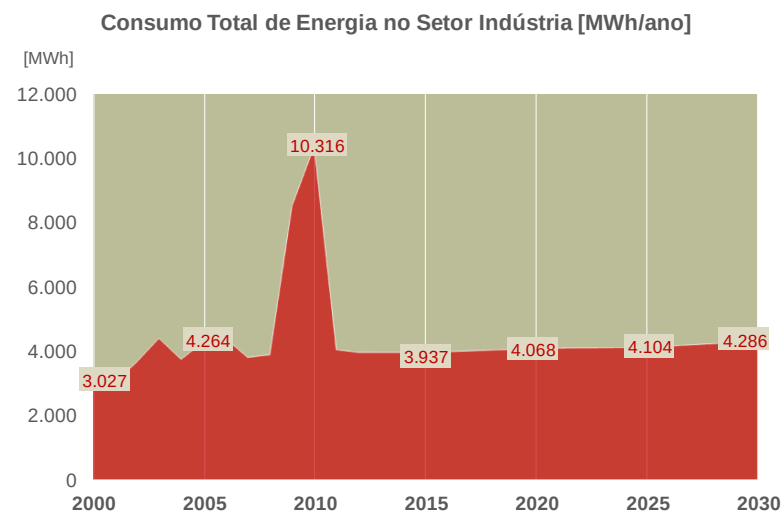
Figura 13 - Consumo Total de Energia no Setor Indústria
