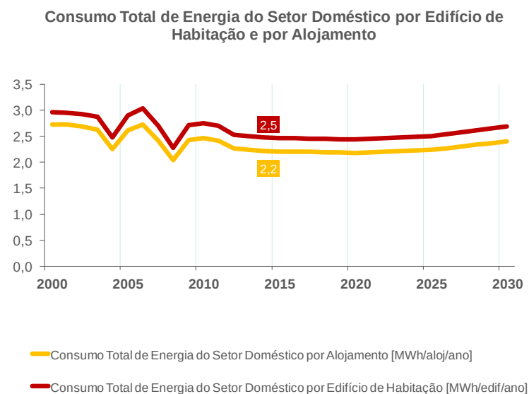
Figura 34 - Consumo Total de Energia do Setor Doméstico por Edifício de Habitação e por Alojamento
