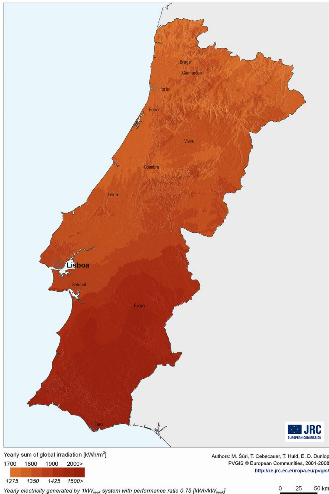
Figura 68 - Irradiação global e potencial máximo de produção de energia elétrica foto voltaica em Portugal Continental (2010) (Fonte: JRC)
