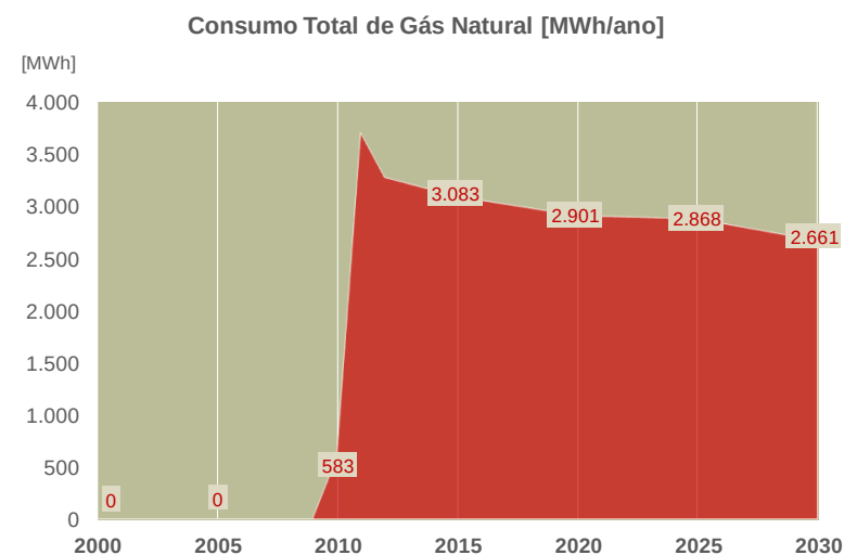
Figura 28 - Consumo Total de Gás Natural
