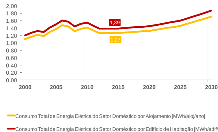
Figura 34 - Consumo Total de Energia Elétrica do Setor Doméstico por Edifício de Habitação e por Alojamento
