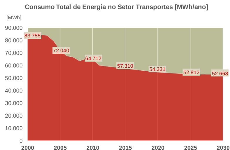
Figura 16 - Consumo Total de Energia no Setor Transportes
