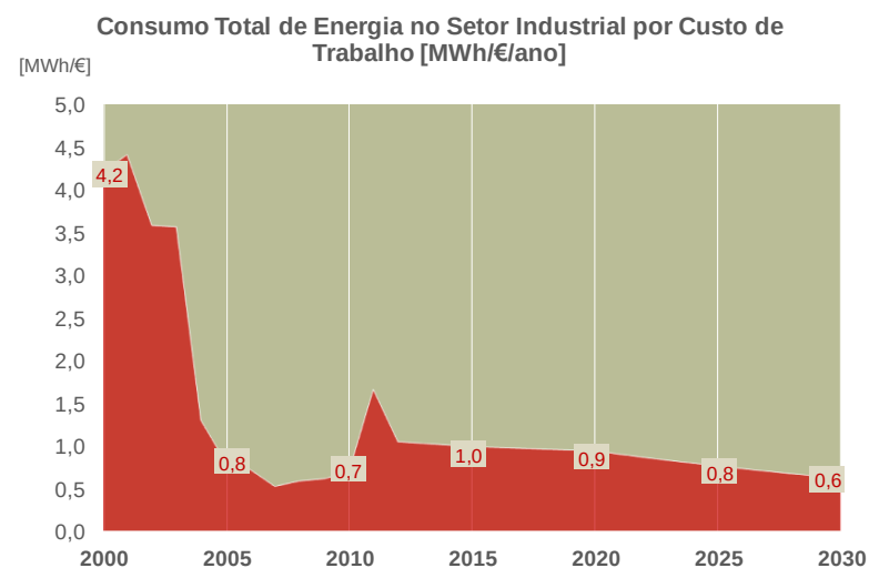
Figura 41 - Consumo Total de Energia no Setor Industrial por Custo de Trabalho
