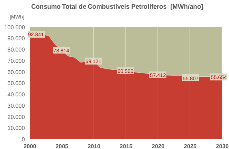
Figura 32 - Consumo Total de Combustíveis Petrolíferos
