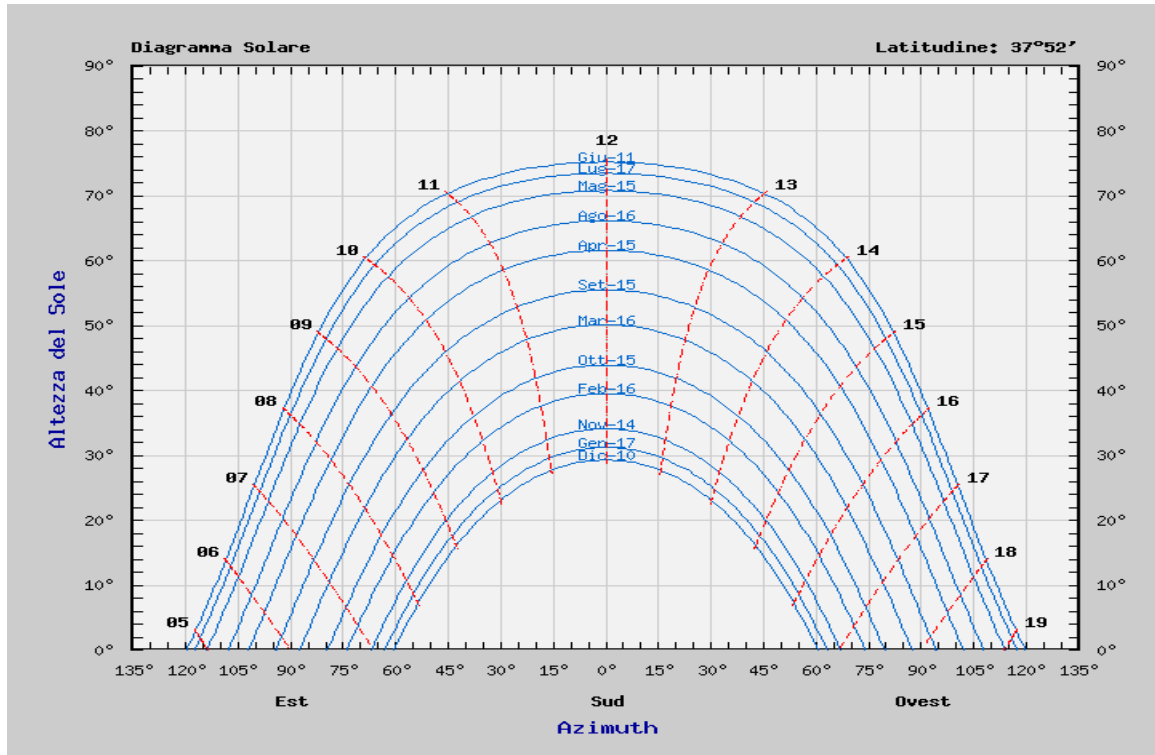
Figura 20. Diagramma solare.
