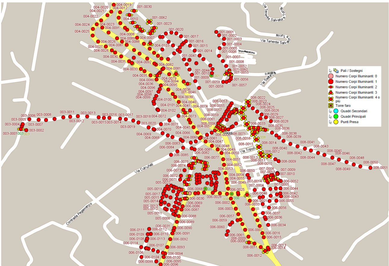
Figura 62. Planimetria Impianto di Pubblica Illuminazione (sezione 1).
