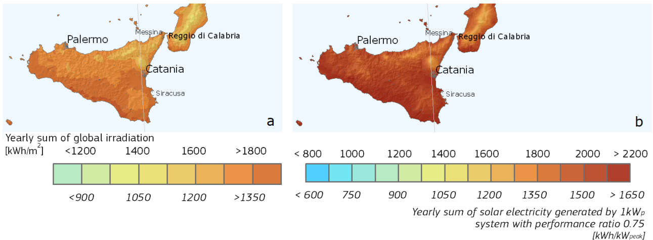
Figura 19. Radiazione solare globale e potenziale elettrico: a) orizzontale; b) angolo ottimale.
