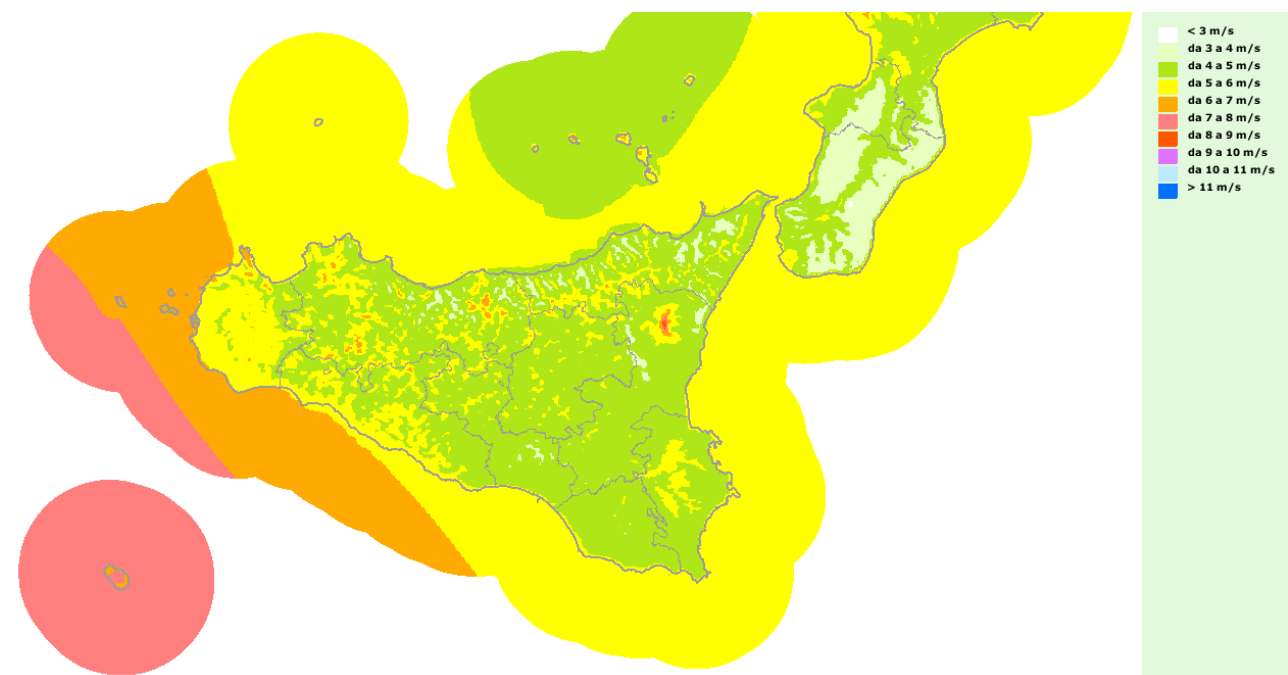
Figura 22. Velocità del vento a 25 metri s.l.m..
