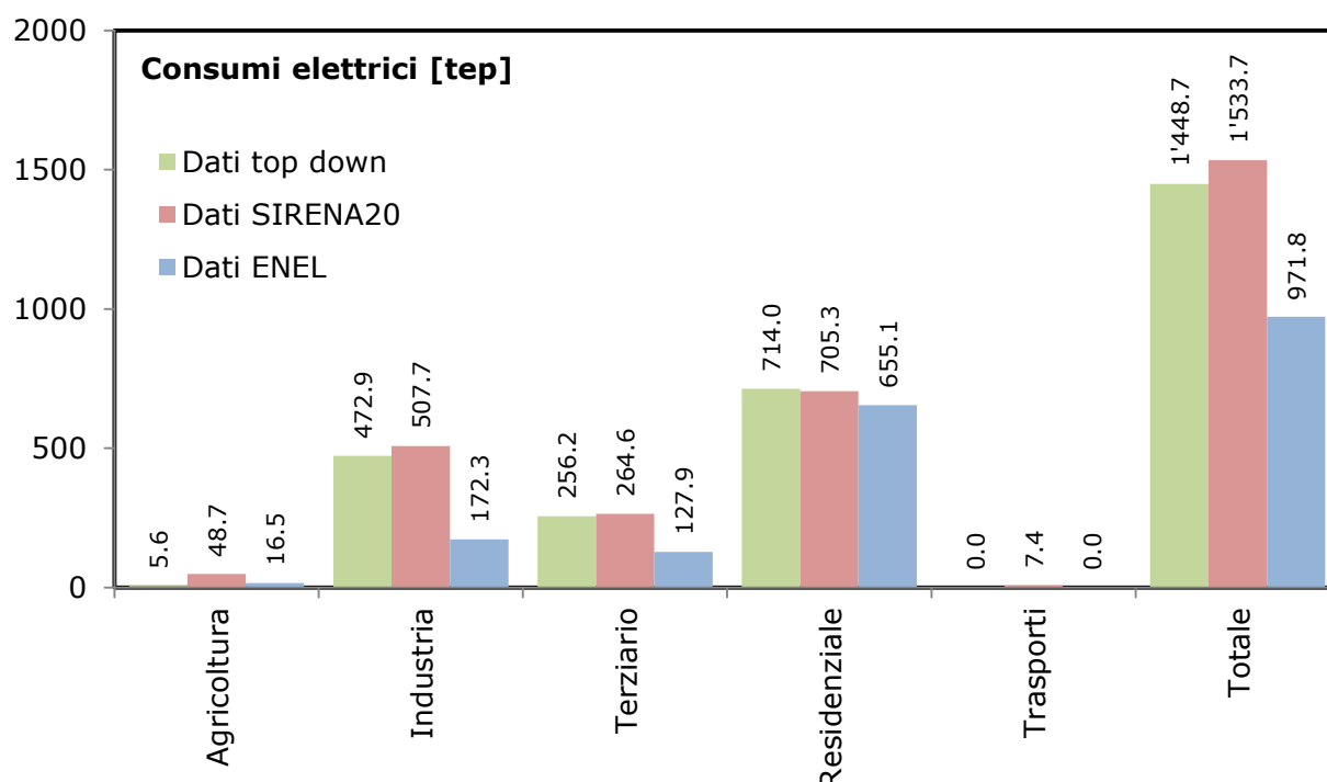
Figura 51. Consumi di energia elettrica del territorio (2011).
