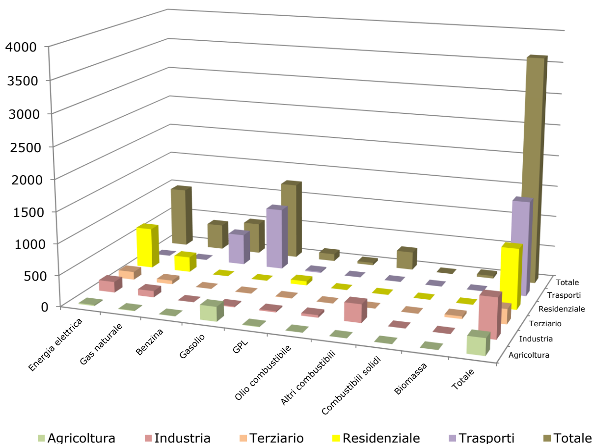
Figura 58. Consumi del territorio (2011).
