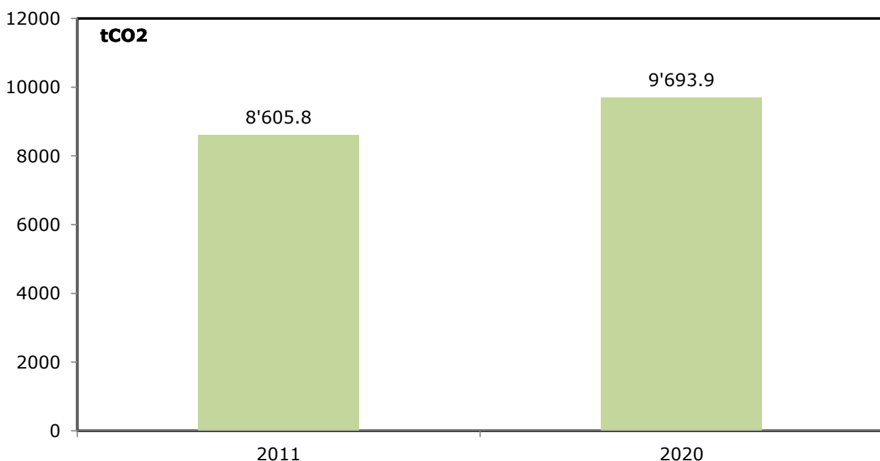
Figura 65. Scenario emissioni di CO 2 senza alcuna politica energetica.
