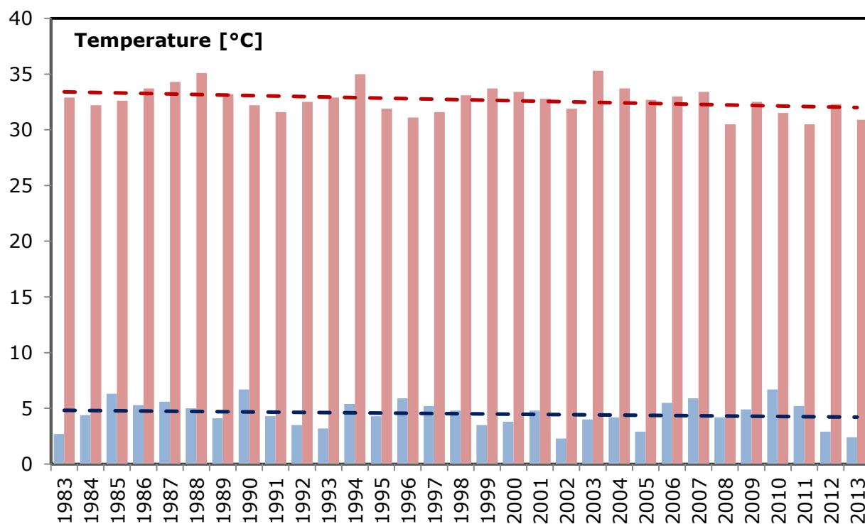
Figura 16. Andamento delle temperature massime e minime (1983-2013).
