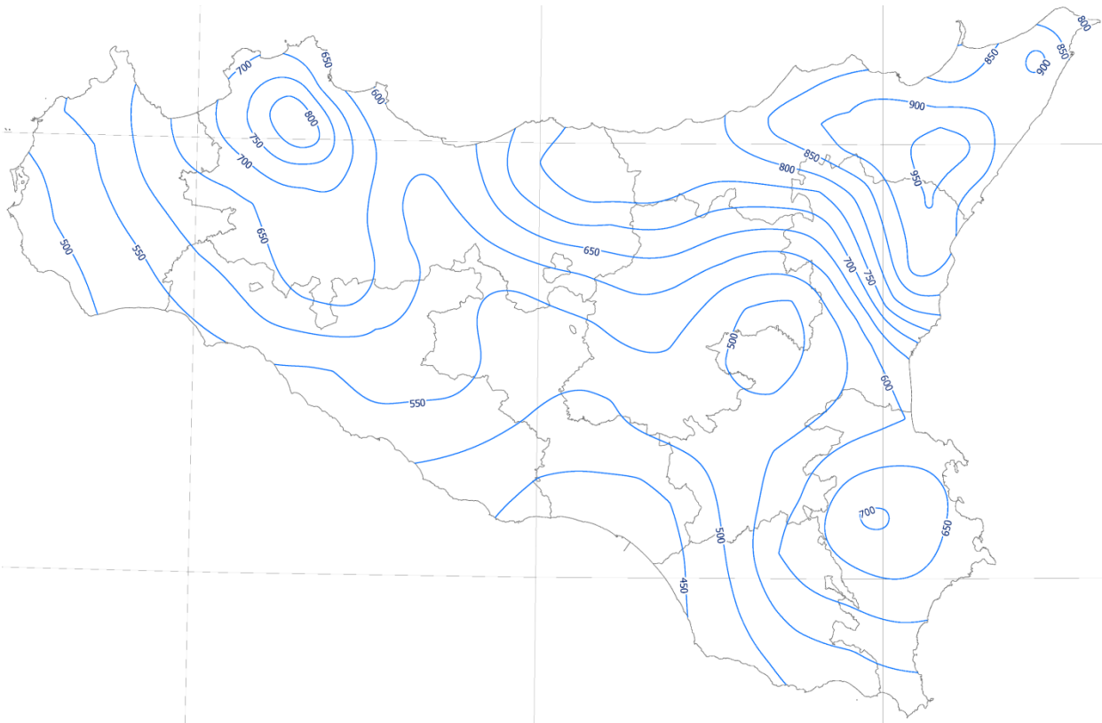
Figura 17. Carta delle isoiete per il periodo dal 1971 al 2003.
