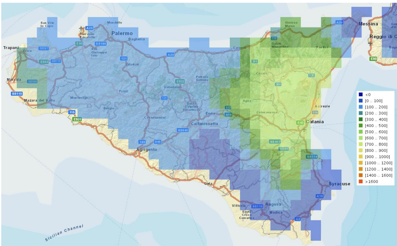
Figura 27. Capacità teorica in PJ/km 2 .
