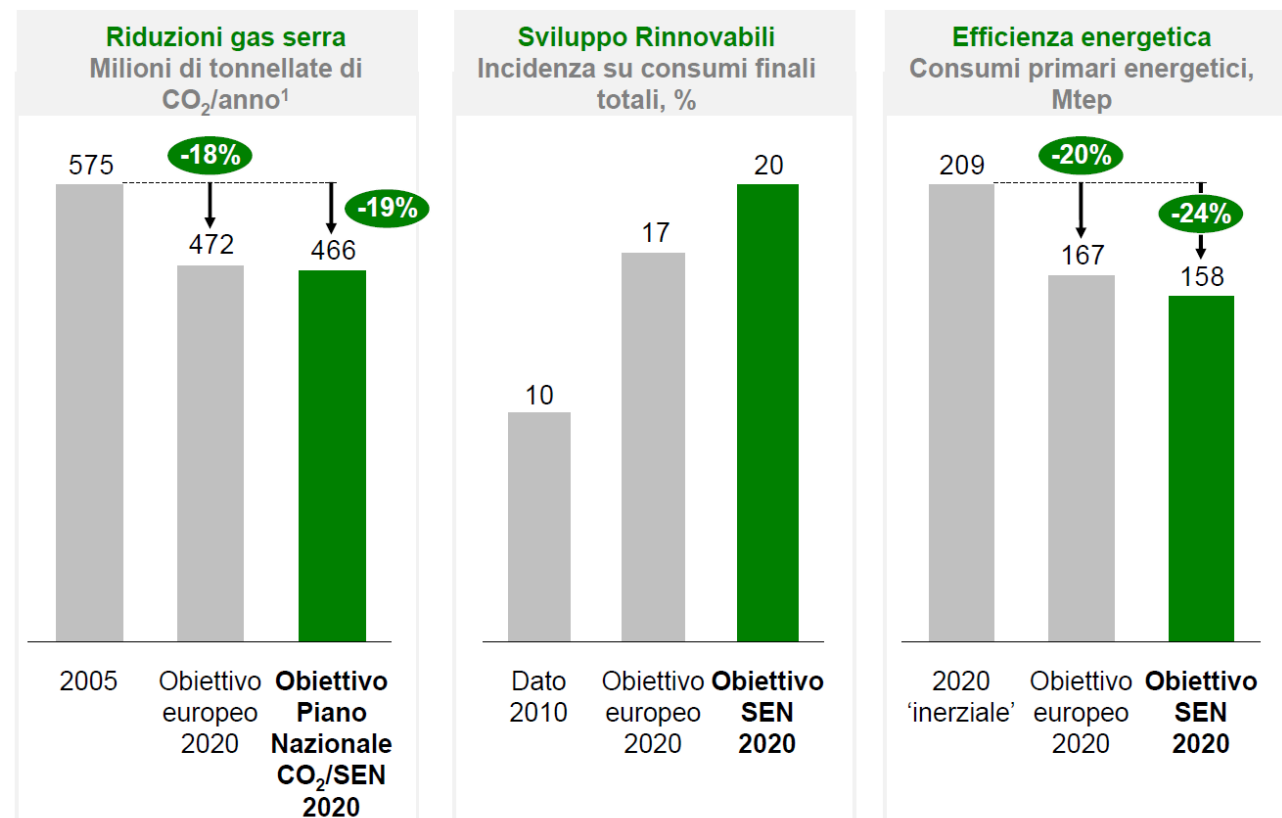
Figura 7. Obiettivi ambientali e di decarbonizzazione.
