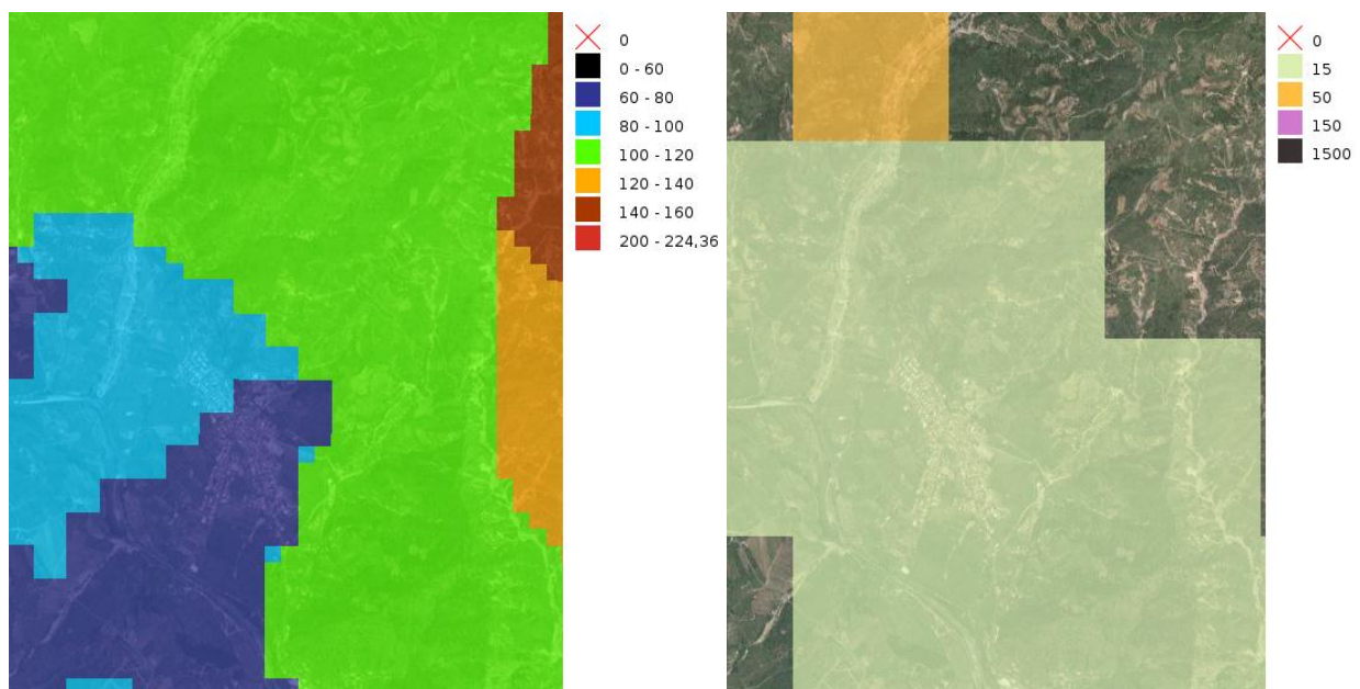
Figura 29. sx) Energia specifica scambiata con il terreno [kWh/m²]; dx) Fabbisogno di calore [TJ/kmq].
