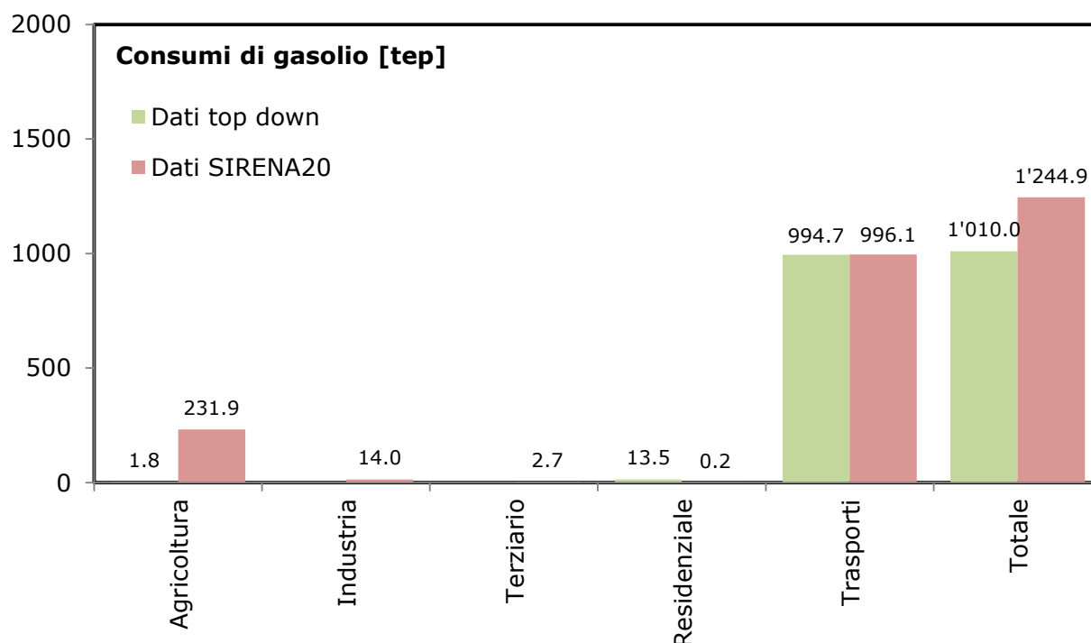
Figura 54. Consumi di gasolio del territorio (2011).
