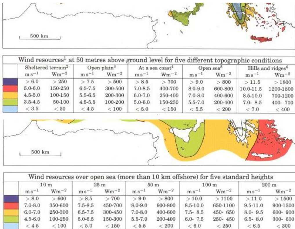
Figura 21. Velocità del vento a 50 metri s.l.m.: a) su suolo; b) off-shore.
