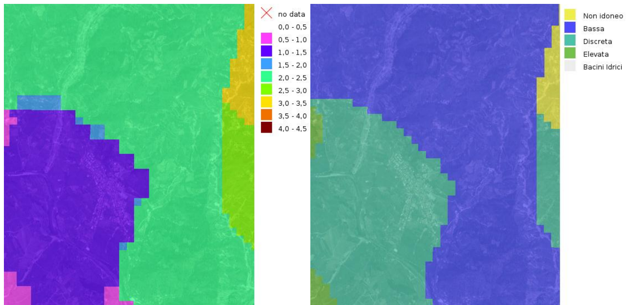
Figura 28. sx) Conducibilità termica calcolata [W/mK]; dx) Idoneità all'utilizzo di sistemi a circuito aperto.
