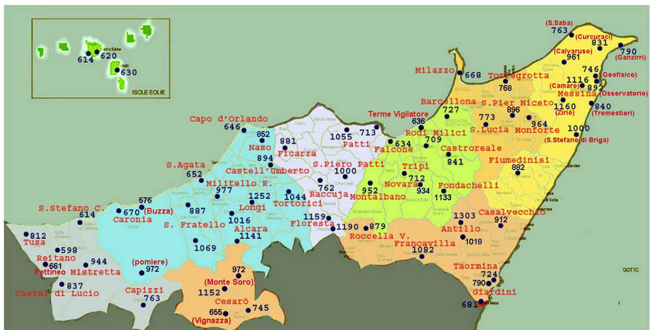
Figura 13. Regime pluviometrico della provincia di Messina.
