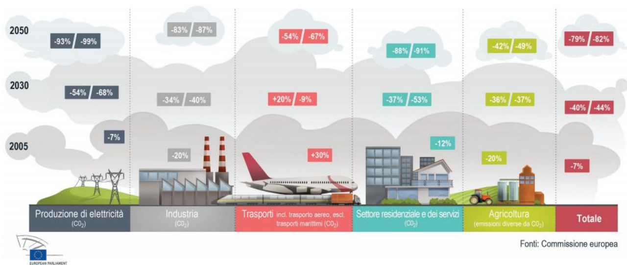
Figura 5. 2050: la strategia per ridurre le emissioni di carbonio - Riduzione dei gas serra rispetto al 1990.
