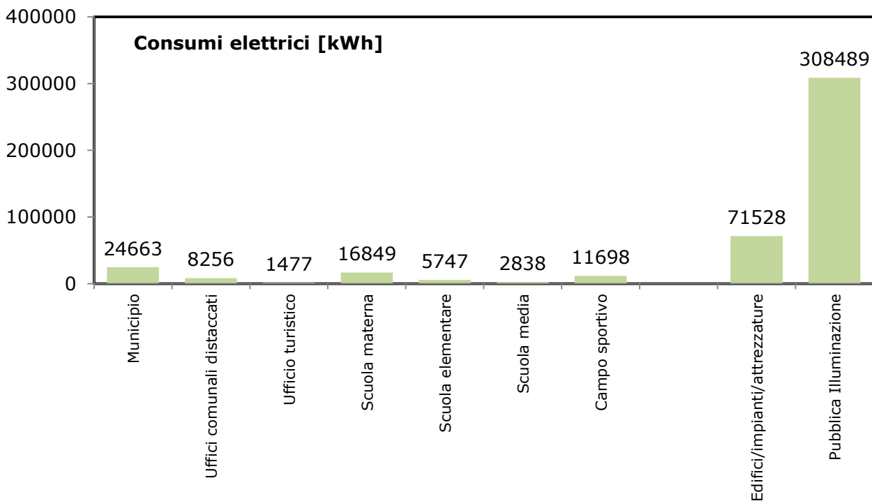
Figura 63. Consumi elettrici comprensivi della pubblica illuminazione (2011).
