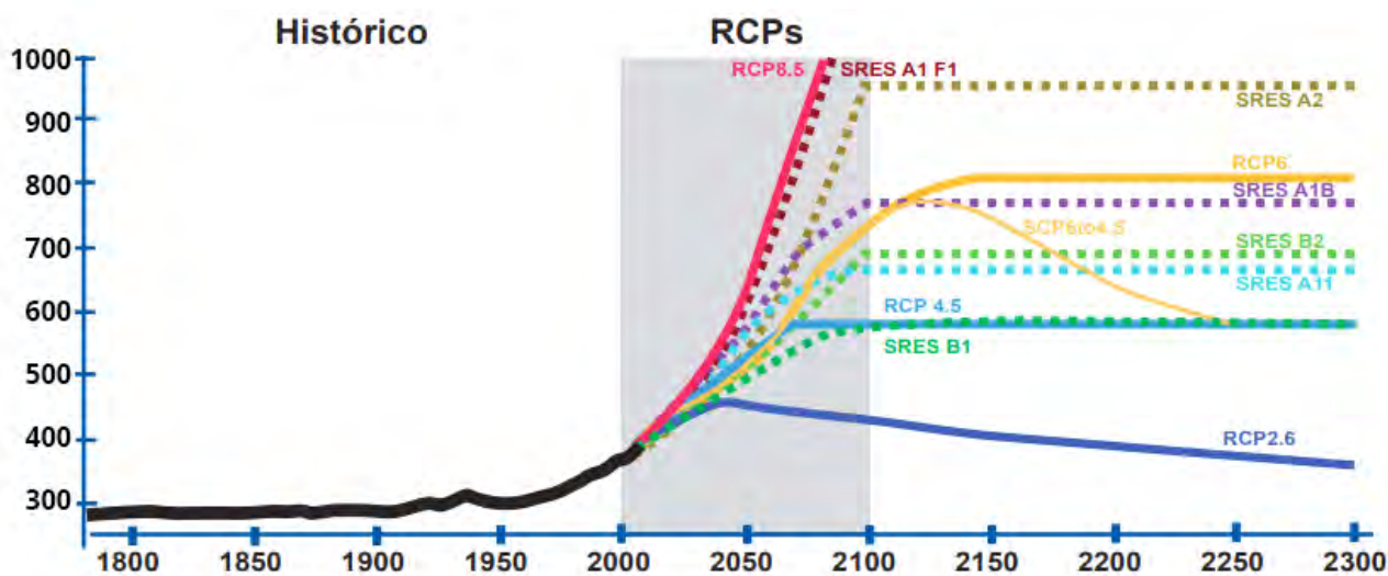
Gráfico 16.- Evolución da concentración de CO 2 equivalente para os distintos escenarios de emisión SRES e RCP. Fonte: MAGRAMA, 2013.
