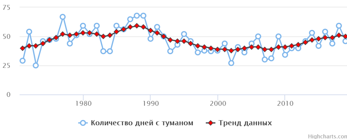
Рисунок 43. График изменения количества дней с туманом с 1971 по 2019 гг.
