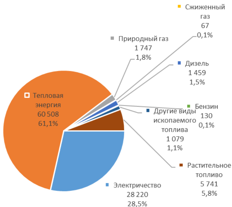
Рисунок 15. Структура выбросов CO 2 муниципальным сектором
