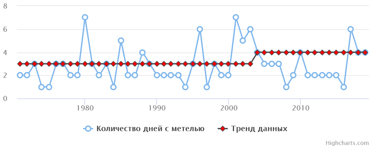
Рисунок 44. График изменения количества дней с метелью с 1971 по 2019 гг.
