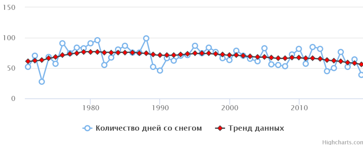
Рисунок 42. График изменения количества дней со снегом с 1971 по 2019 гг.
