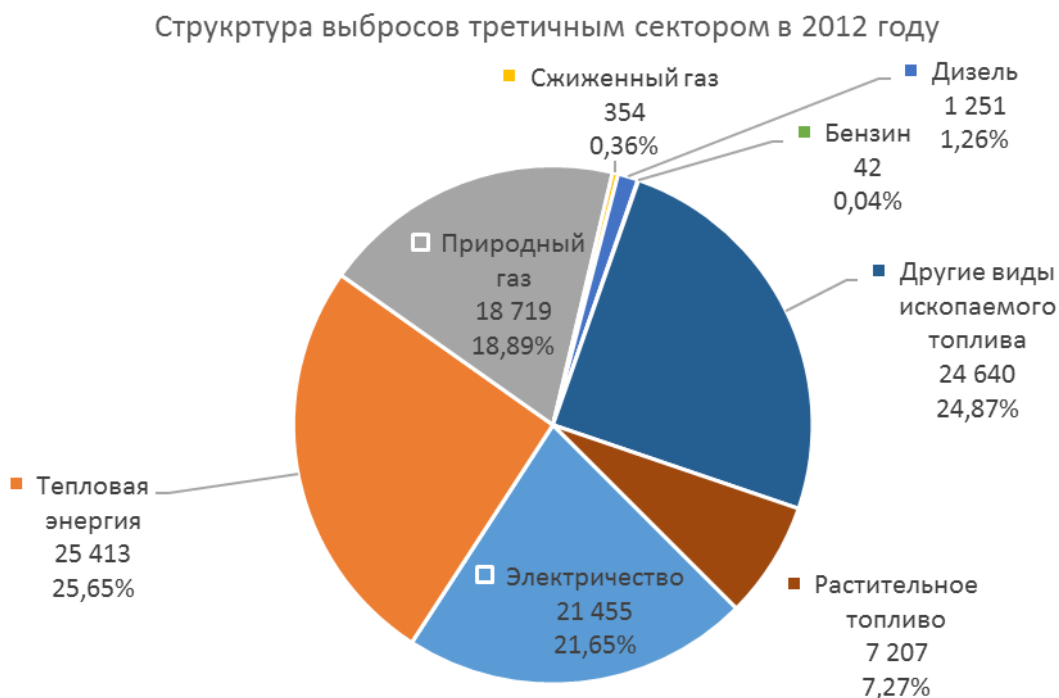
Рисунок 17. Структура выбросов CO 2 третичным сектором, т. CO 2
