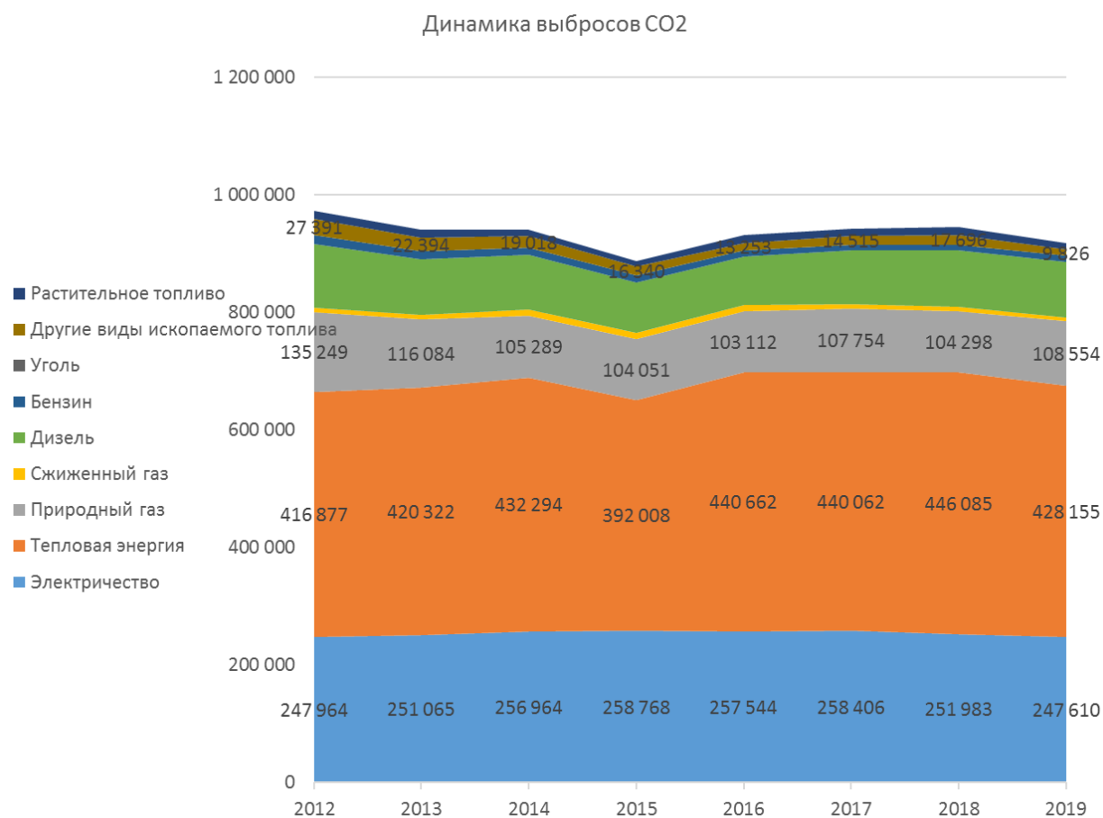
Рисунок 19. Динамика выбросов CO 2
