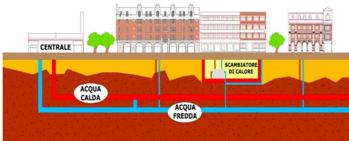
Figura 29: Schema per un impianto di teleriscaldamento
