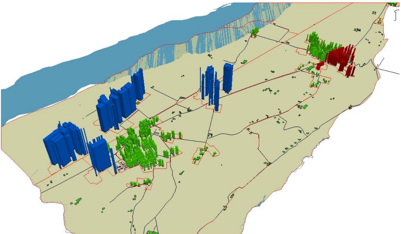
Figura 20: Particolare dei consumi termici nel centro di Ozzano; dati stimati da modello.
