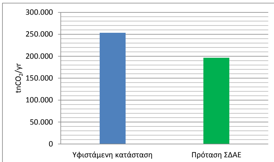
Γράφημα 1: Αναμενόμενα αποτελέσματα των δράσεων του Δήμου Αγίας Παρασκευής
