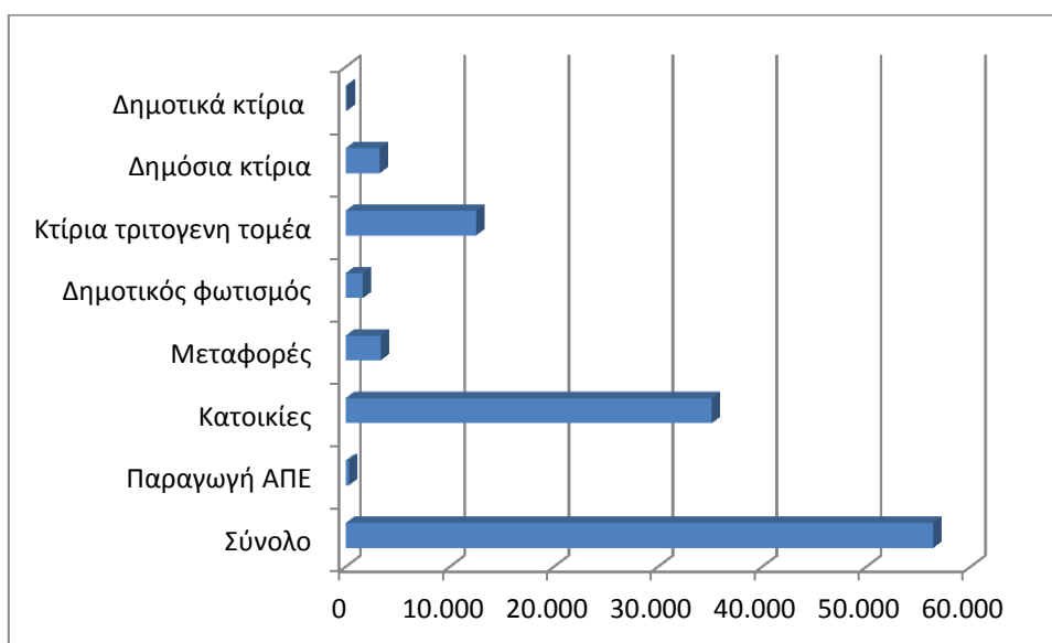
Γράφημα 26: Συμβολή κάθε δράσης στα συνολικά αναμενόμενα αποτελέσματα των δράσεων του Δήμου Αγίας Παρασκευής (μείωση εκπομπών σε tCO 2 /έτος)
