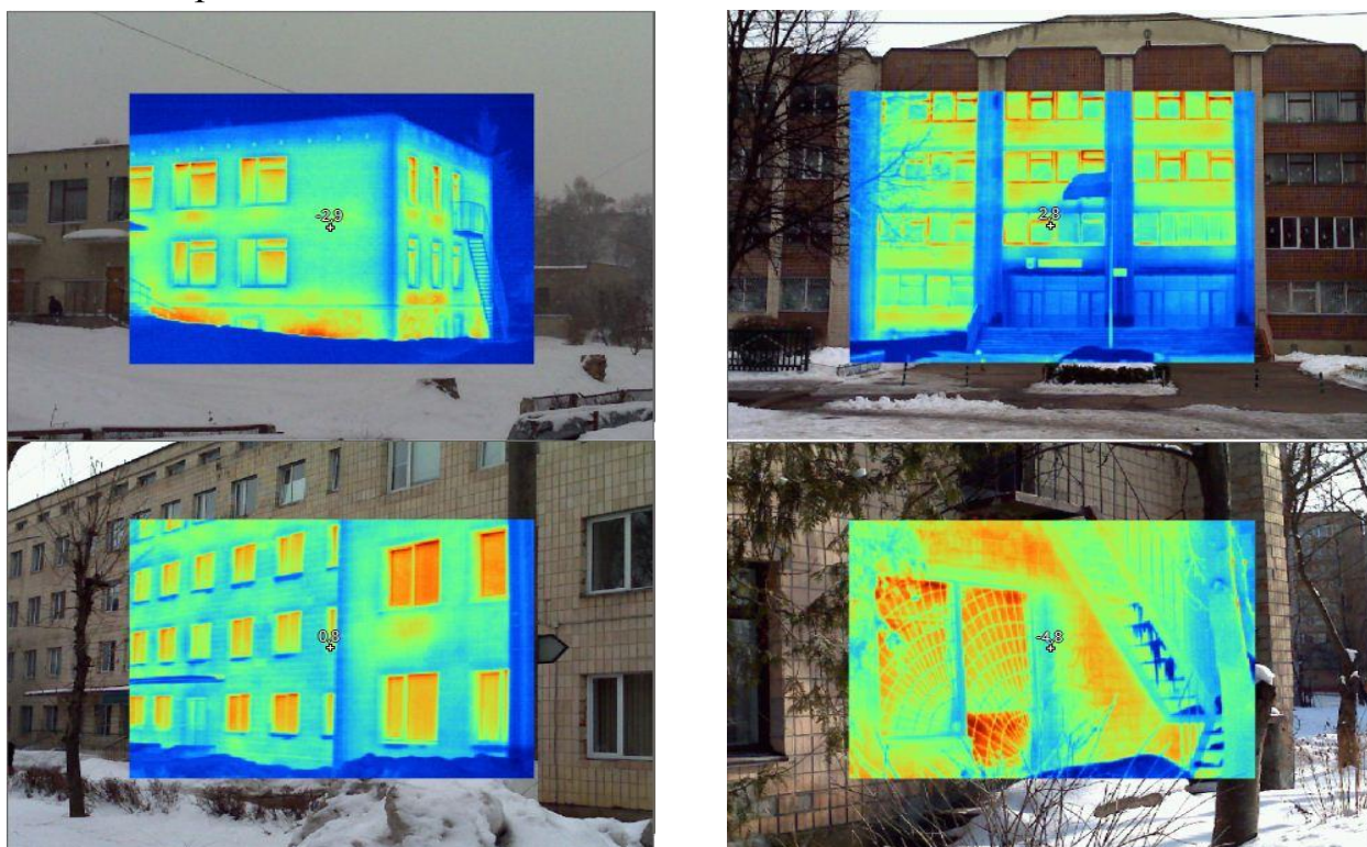
Рис. 2.2.1.1. Тепловізійне обстеження огорожувальних конструкцій будівель бюджетної сфери, що фінансуються з міського бюджету м. Тернопіль
