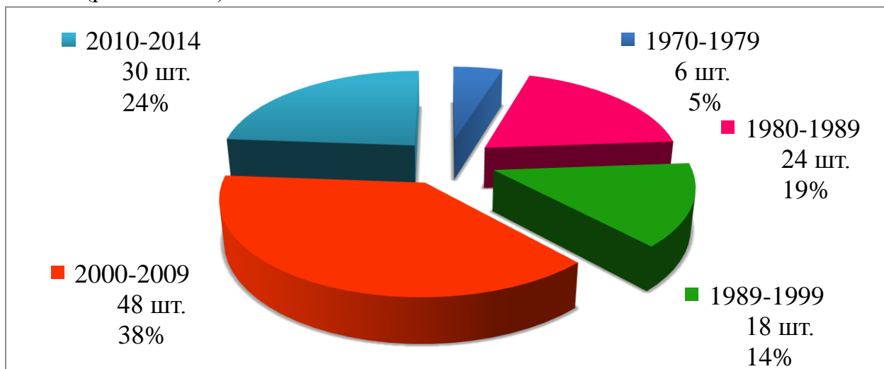
Рис. 2.1.1.1. Роки встановлення та кількість котлів на котельнях в м. Тернопіль
