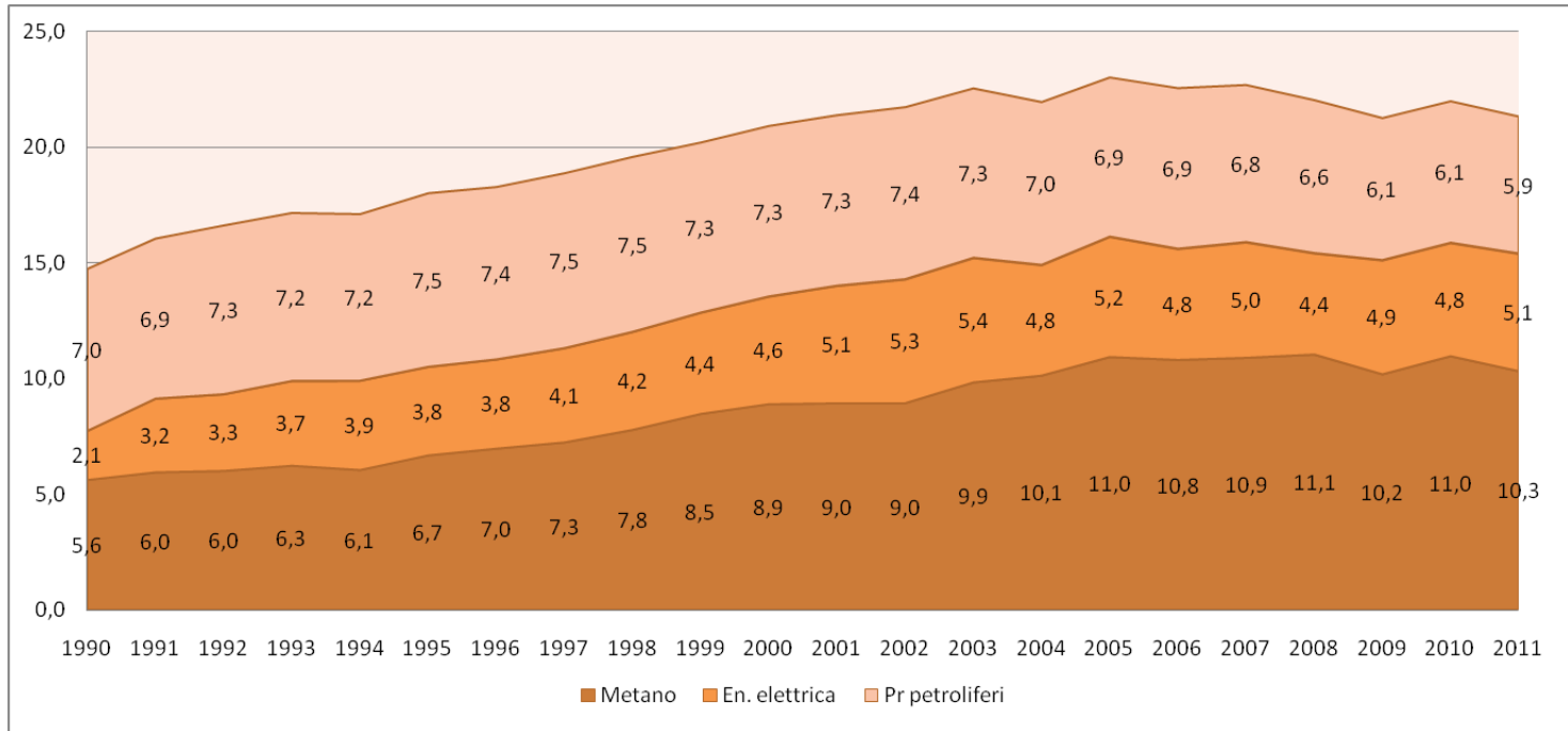
Figura 05 – andamento generale dei consumi [kTep] suddiviso per vettore energetico utilizzato
