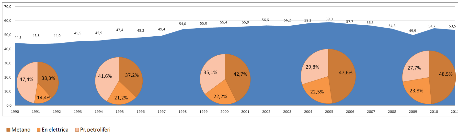
Figura 19: andamento delle emissioni di CO2 (kTon) in funzione dei diversi vettori energetici
