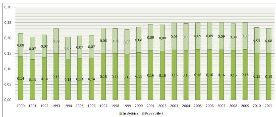
Figura 06: Uso di pr. petroliferi ed energia elettrica in Agricoltura (kTep)
