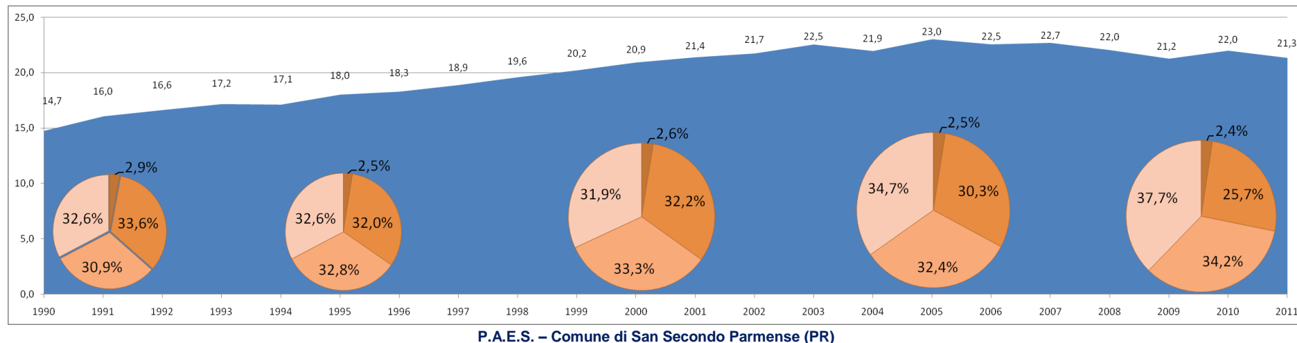
Figura 04 – andamento generale dei consumi (kTep) e dettaglio per settore per gli anni 1990, 1995, 2000, 2005, 2011
