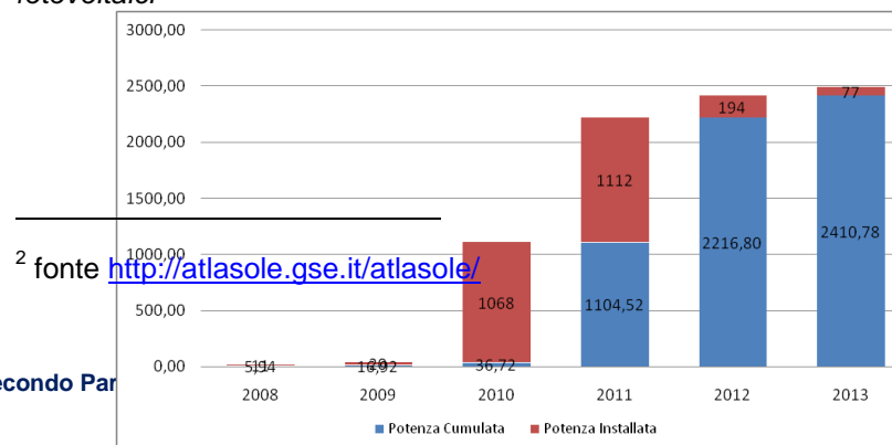
Figura 14: potenza installata annualmente e cumulata [kW] di imp. fotovoltaici
