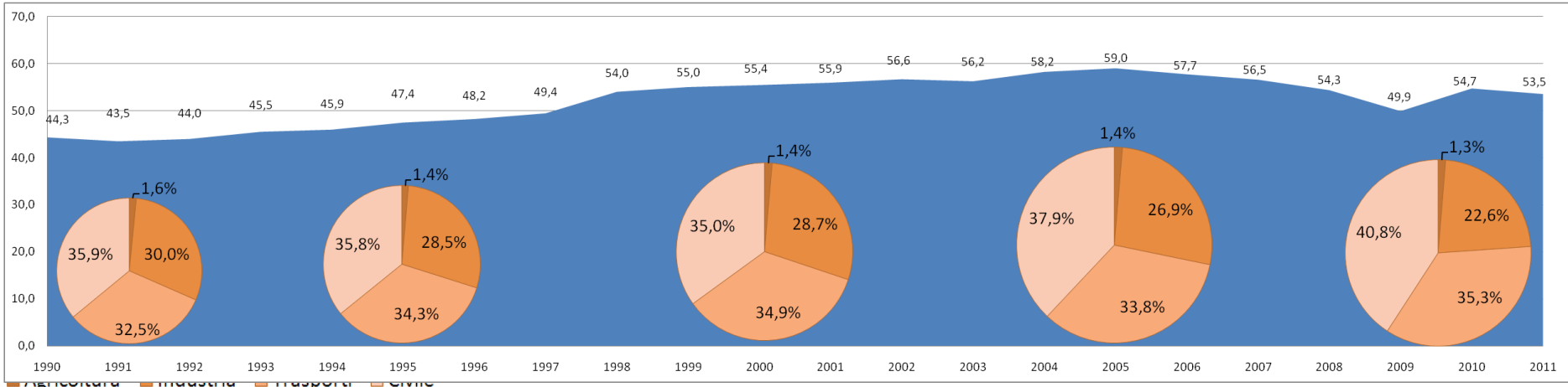
Figura 20: andamento delle emissioni di CO2 (kTon) in funzione dei diversi settori socio-economici
