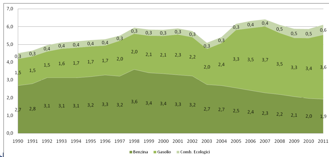
Figura 12: andamento dei consumi [kTep] per vettore energetico
