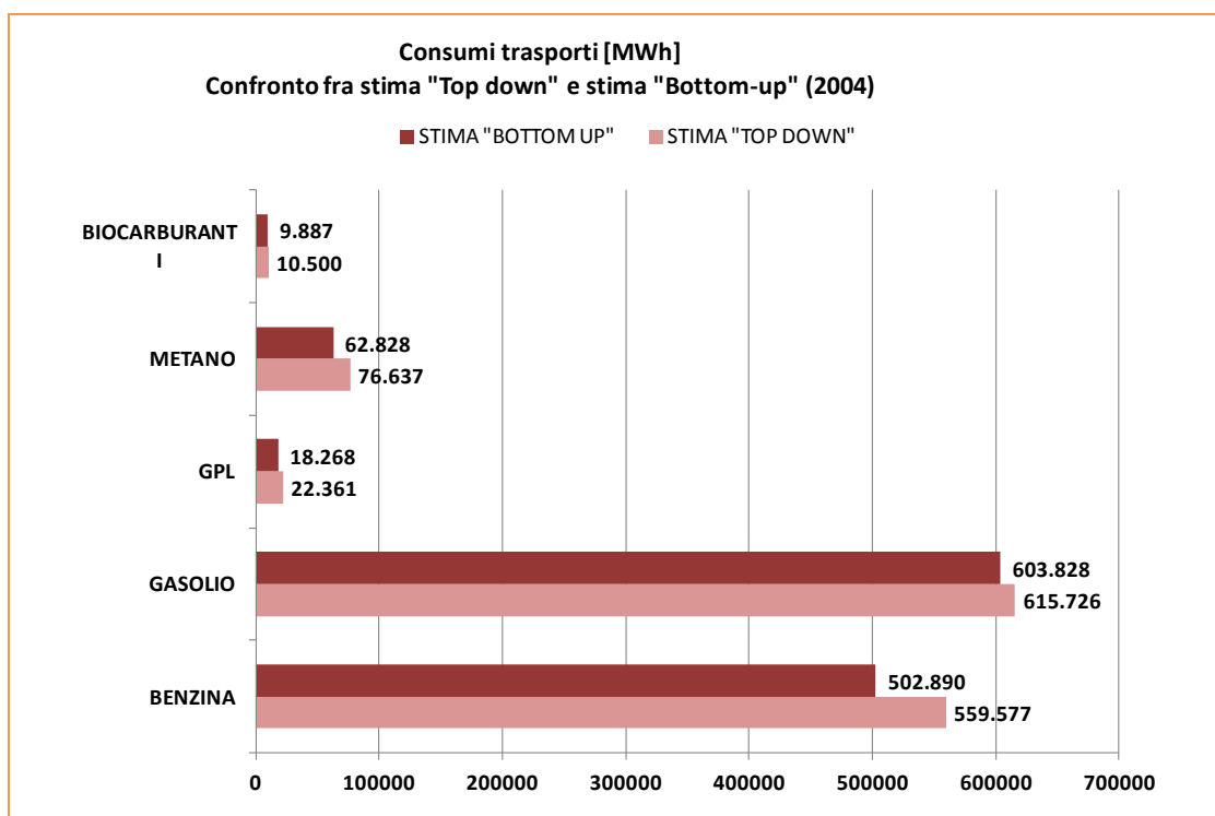
Figura 4-8– Confronto fra la stima “top down” e la stima “bottom-up” per i consumi di carburanti nel settore trasporti nel Comune di Parma, anno 2014 (fonte: Ministero dello Sviluppo Economico, dati ACI, elaborazione La Esco del Sole)
