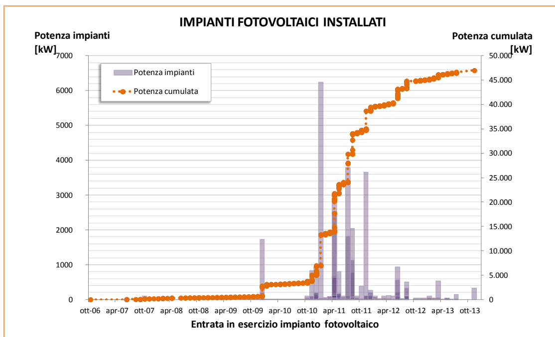
Figura 3-8 – Potenza cumulata degli impianti fotovoltaici installati nel Comune di Parma, dati dal 2007 al 2012 (Fonte: ATLASOLE – elaborazione La Esco del Sole)
