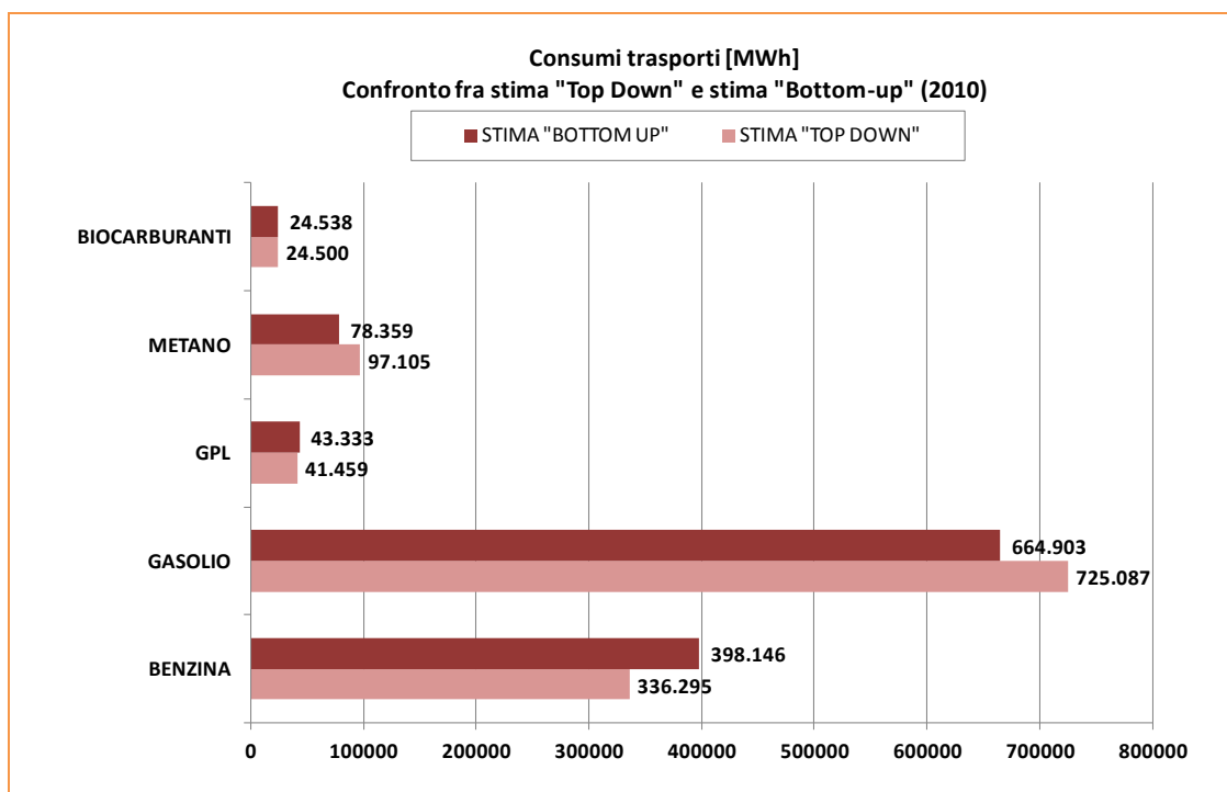
Figura 4-9– Confronto fra la stima “top down” e la stima “bottom-up” per i consumi di carburanti nel settore trasporti nel Comune di Parma, anno 2010 (fonte: Ministero dello Sviluppo Economico, dati ACI, elaborazione La Esco del Sole)
