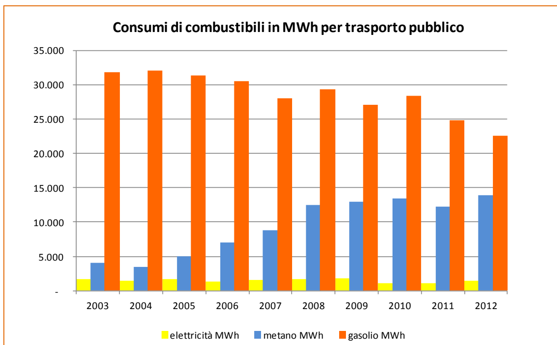
Figura 4-1 – Consumi di gasolio, gas metano ed energia elettrica per trasporto pubblico nel Comune di Parma in MWh (Fonte: TEP Spa, elaborazione La ESCo del Sole).
